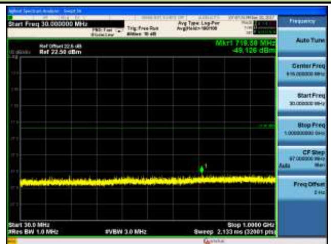
802.11n-40M CH06 (2437MHz)
