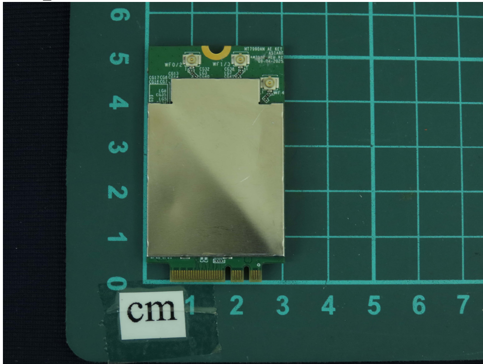
(1) EUT Photo_M/N: AW7990-AED
