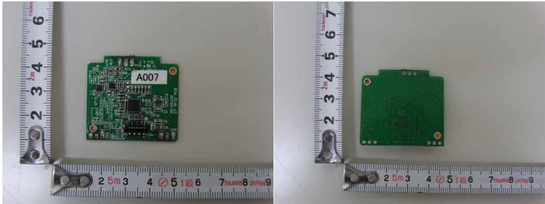
RF module
