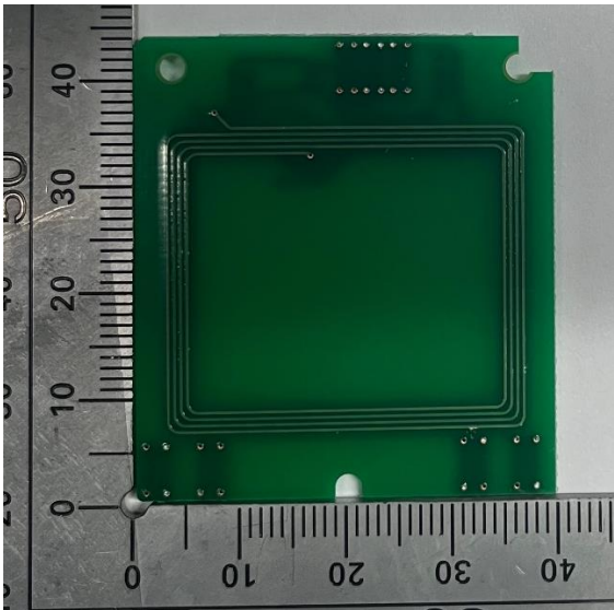
Antenna
