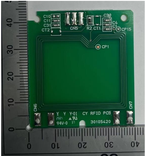
Antenna
