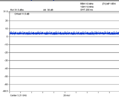
802.11ac (VHT80)
