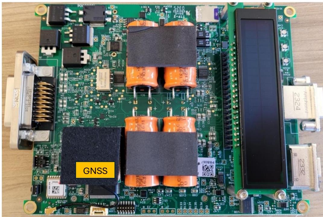
PCB Top
