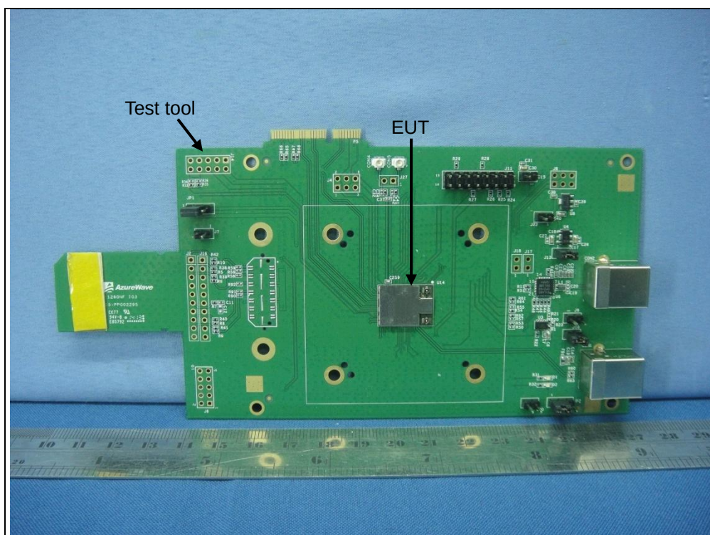
EUT + Test tool
