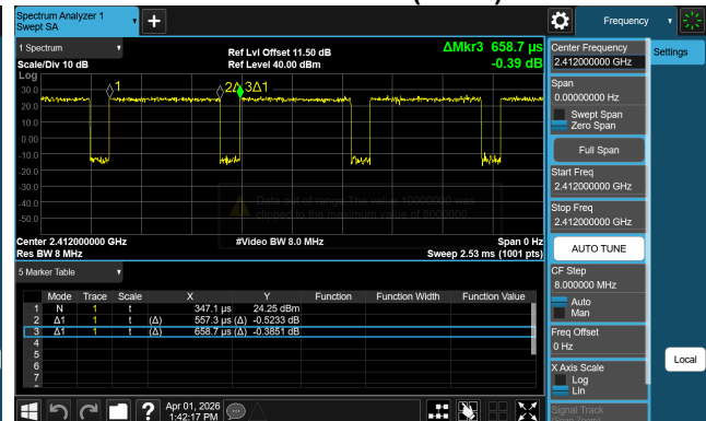
IEEE 802.11ax(HE20)
