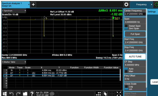
IEEE 802.11b
