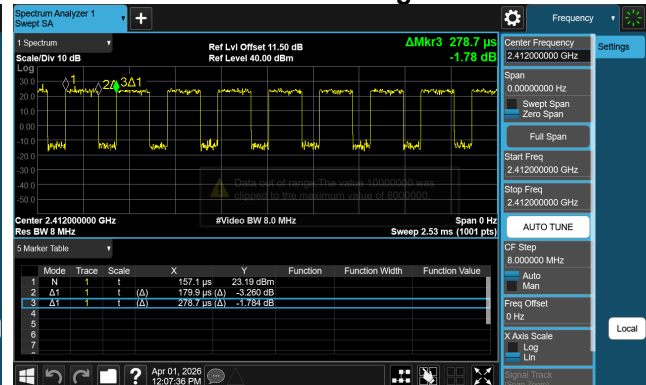
IEEE 802.11g
