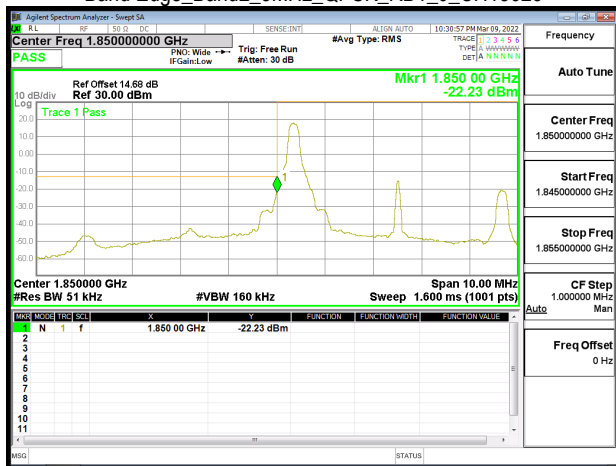
Band Edge_Band2_5MHz_QPSK_RB1_0_CH18625
