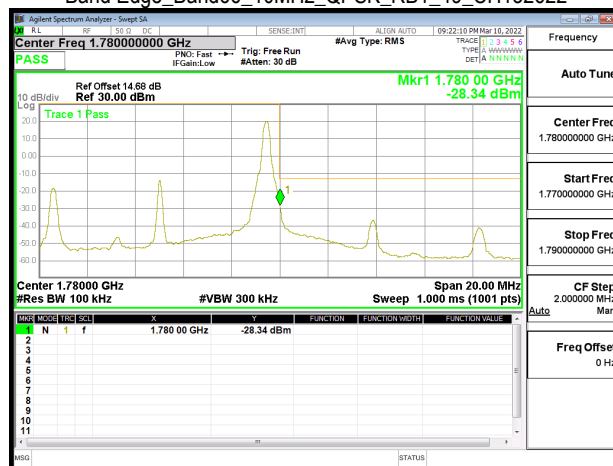
Band Edge_Band66_10MHz_QPSK_RB1_49_CH132622
