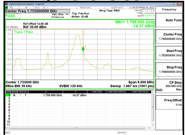
Band Edge_Band4_3MHz_QPSK_RB1_14_CH20385
