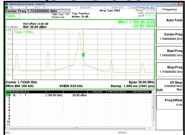
Band Edge_Band4_15MHz_QPSK_RB1_74_CH20325
