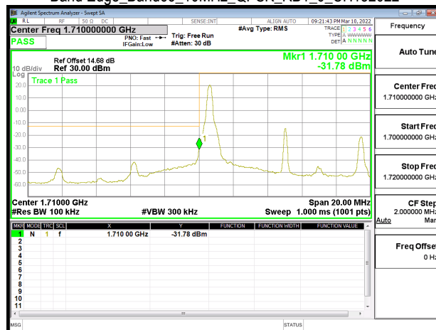
Band Edge_Band66_10MHz_QPSK_RB1_49_CH132622
