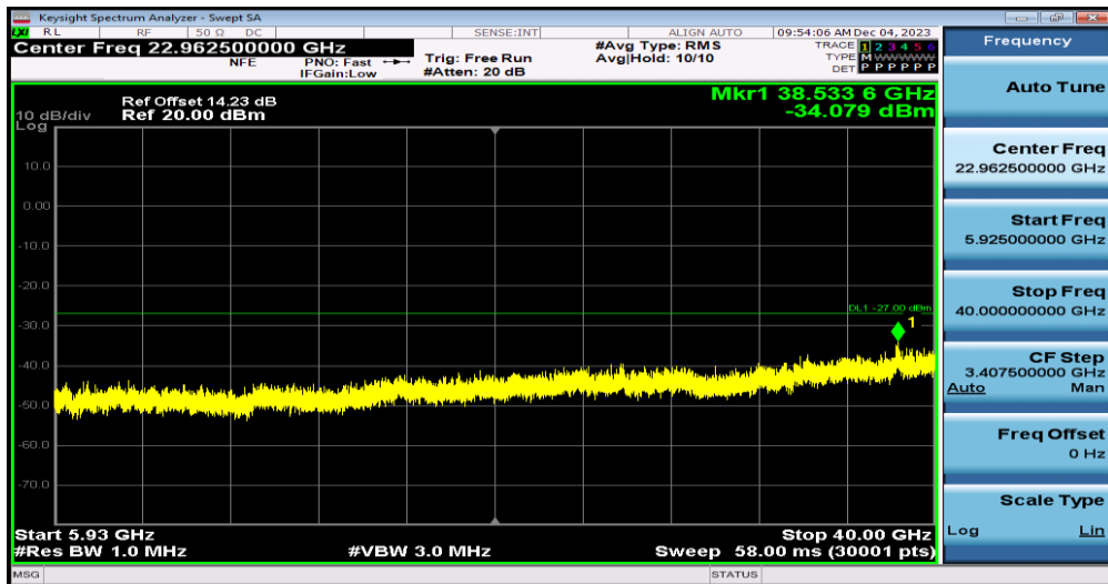
11N40MIMO-Ant0-5755-5925~40000
