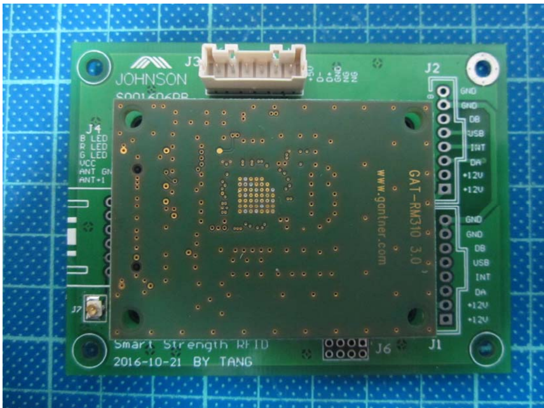
NFC module
