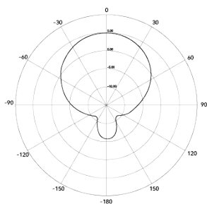
E-Plane HPBW
