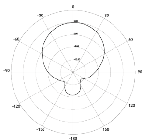
H-Plane HPBW
