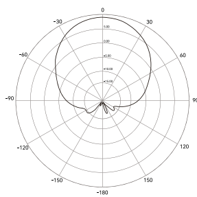
H-Plane HPBW
