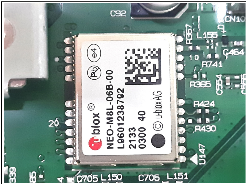
&lt;Module&gt;
