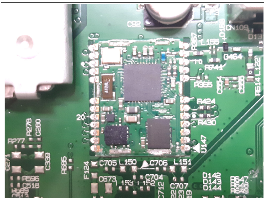
&lt;Module&gt;
