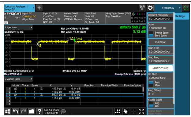
802.11ac(VHT80)
