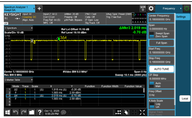
802.11ac(VHT20)
