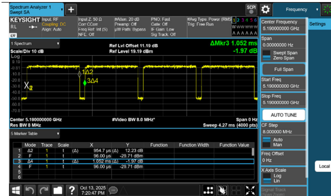
802.11ac(VHT40)
