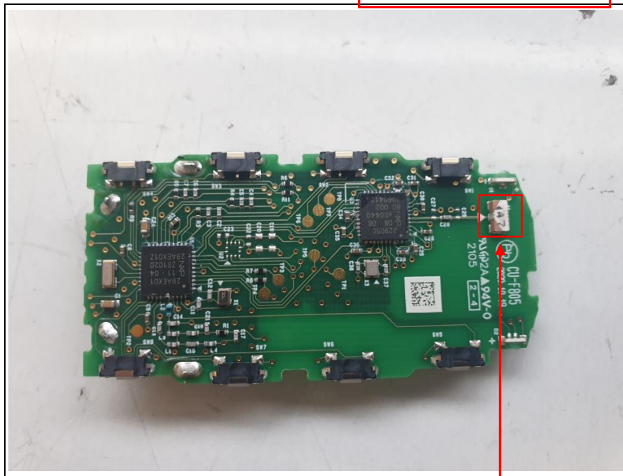
UWB Chip Antenna
