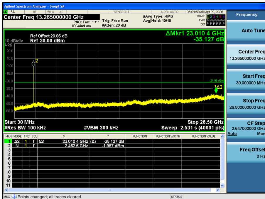
[ANT.2] 802.11n(HT20) - CH 11
