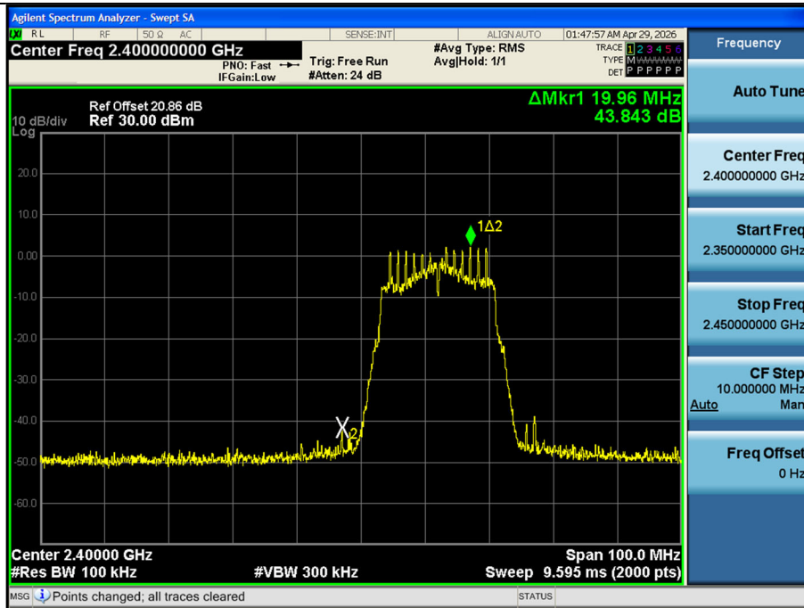
[ANT. 2] 802.11n(HT20) - CH 1
