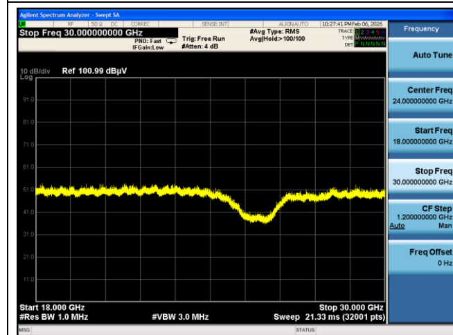
18 GHz ~ 30 GHz
