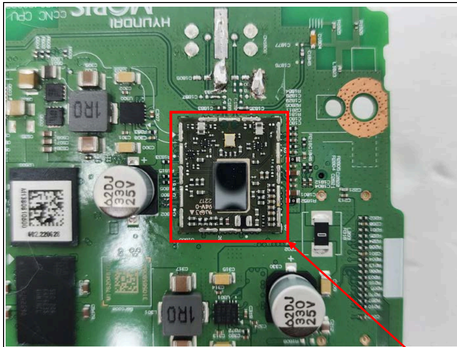
BT/WIFI Module
