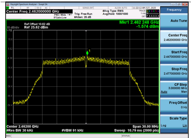
802.11n_HT20-CH 11
