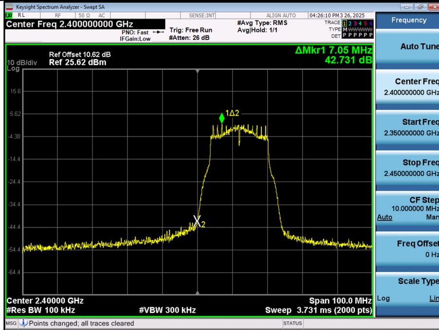
802.11g-CH 1
