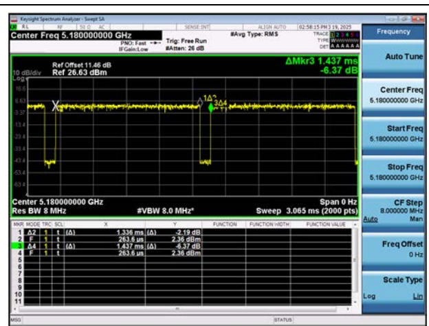
802.11ac(VHT20)
