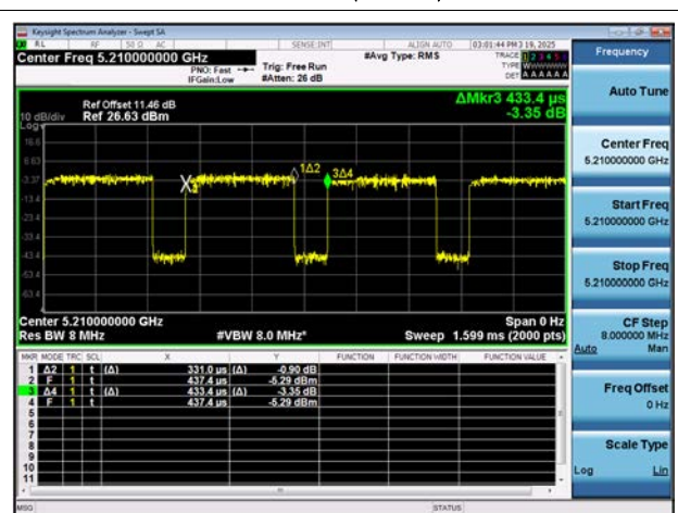
802.11ac(VHT80)
