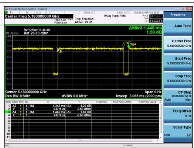
802.11ac(VHT80)
