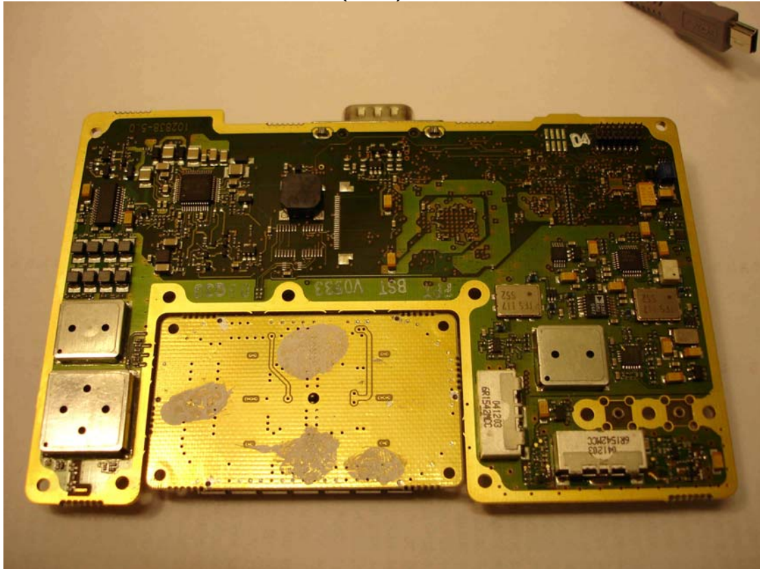
Nera WorldPro 1000 Antenna unit (ODU)
