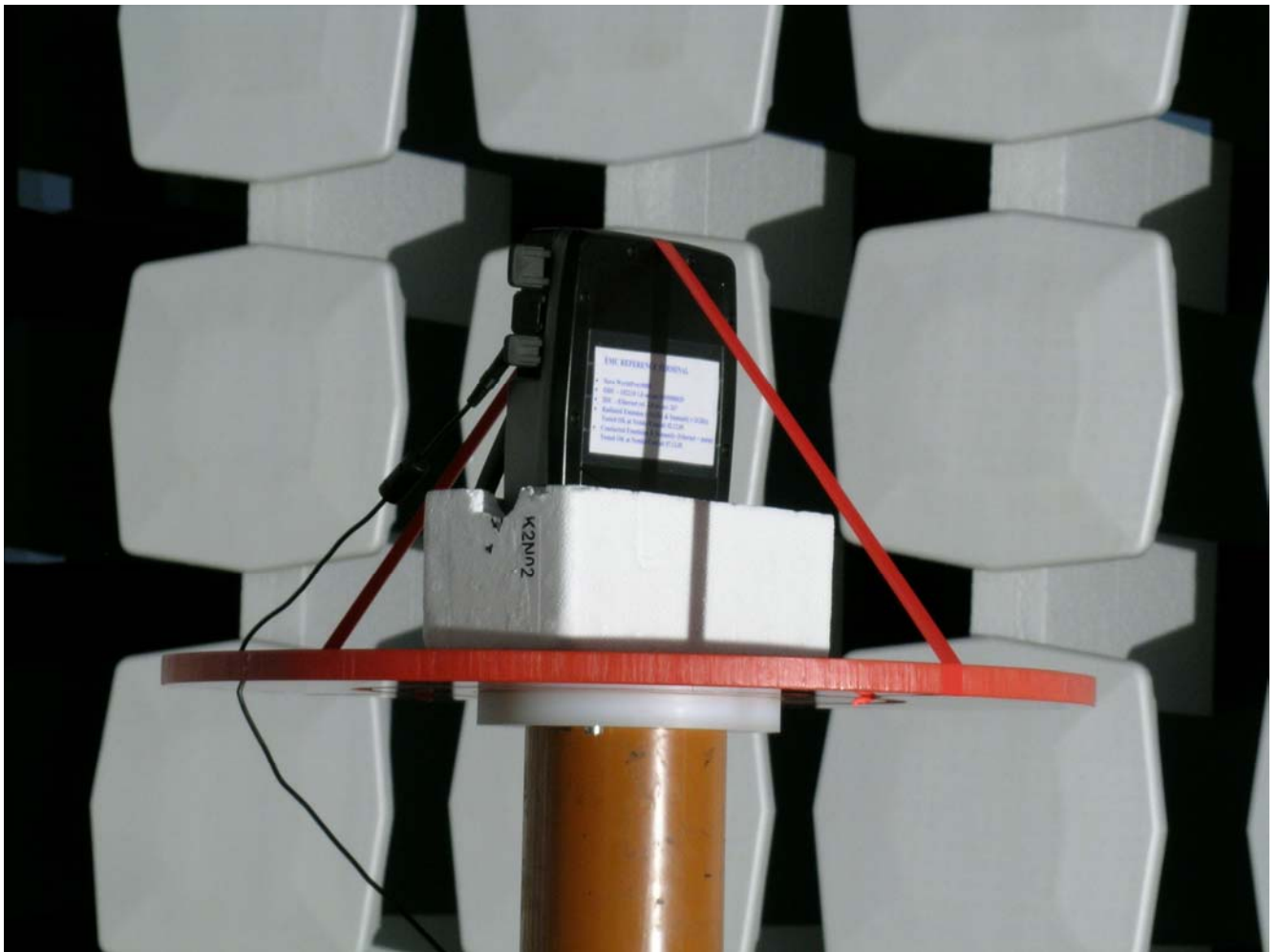
Fig 3 EUT
