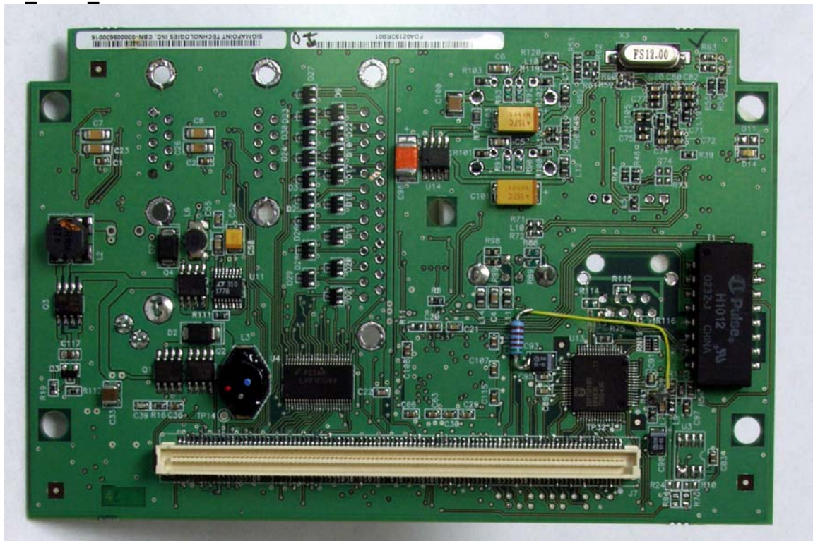
IO_board_2
