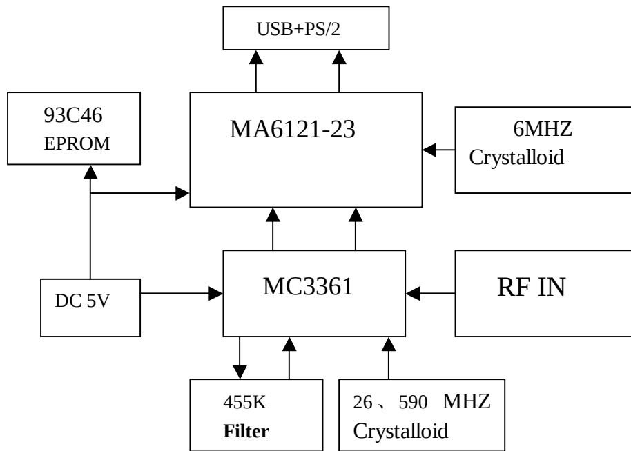
发射方框图
