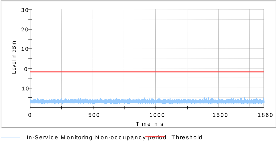
802.11a 5320MHz
