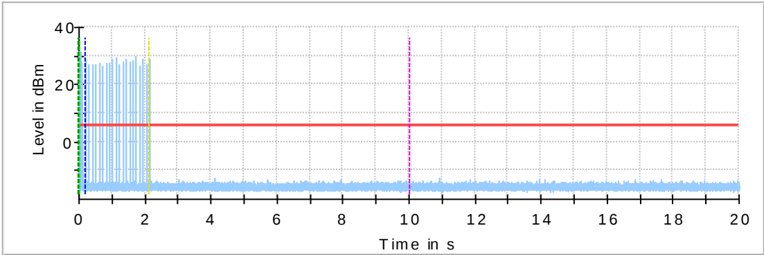
802.11a 5700MHz
