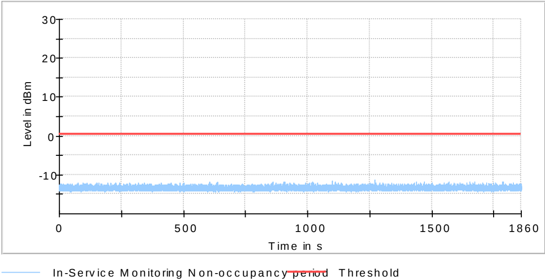
802.11n HT40 5510MHz
