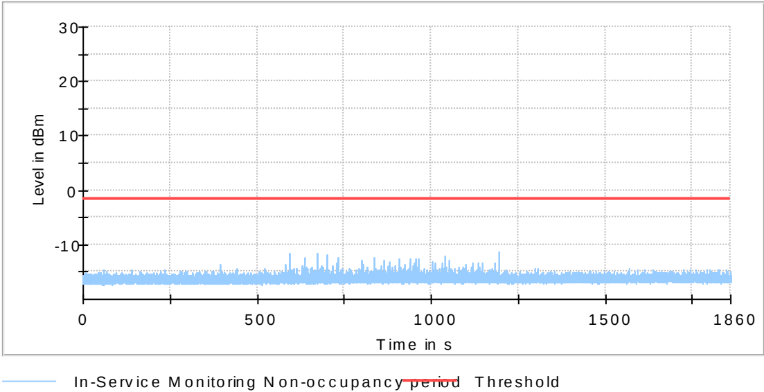
802.11ax HE80 5530MHz
