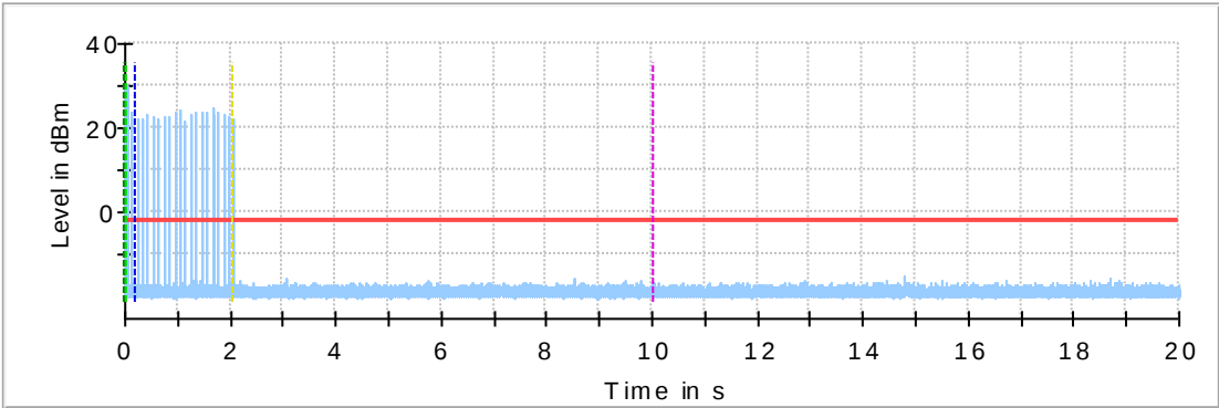
802.11a 5320MHz
