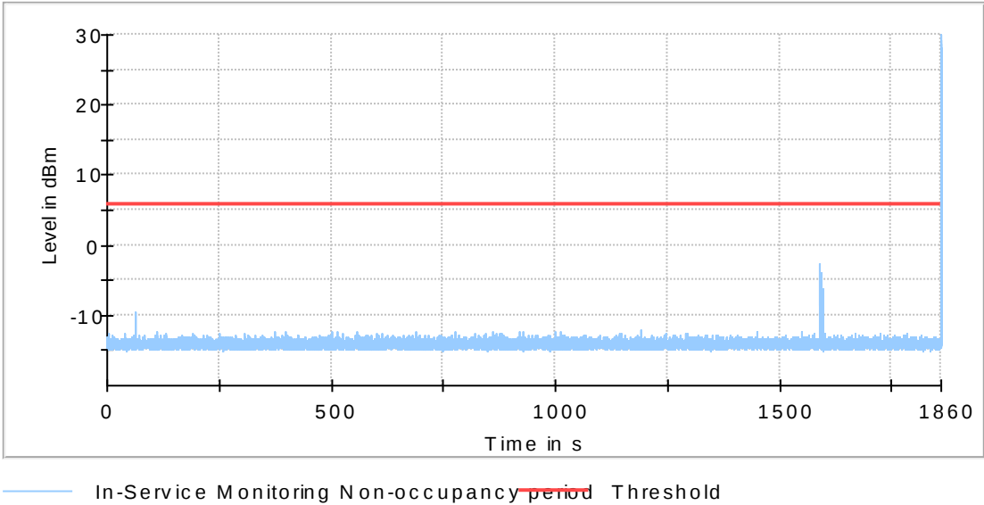
802.11a 5700MHz
