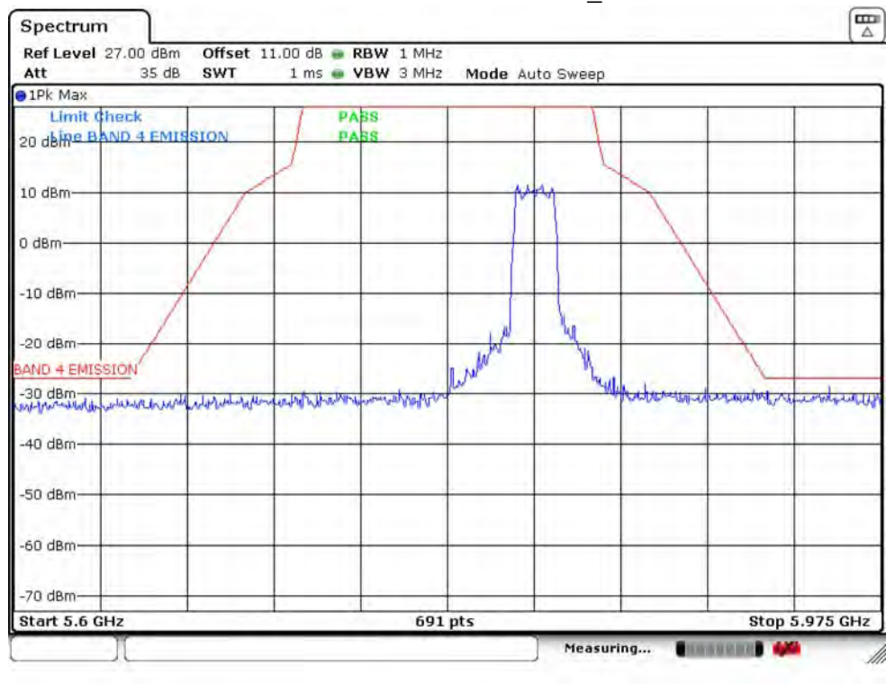
IEEE 802.11n HT20 5825MHz_Ant 2
