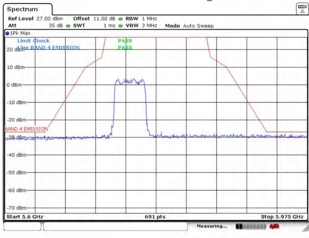
IEEE 802.11ax HE40 5755MHz_Ant 1
