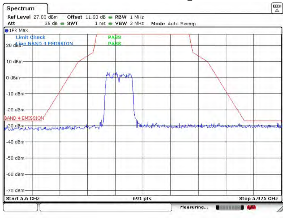
IEEE 802.11n HT40 5755MHz_Ant 1
