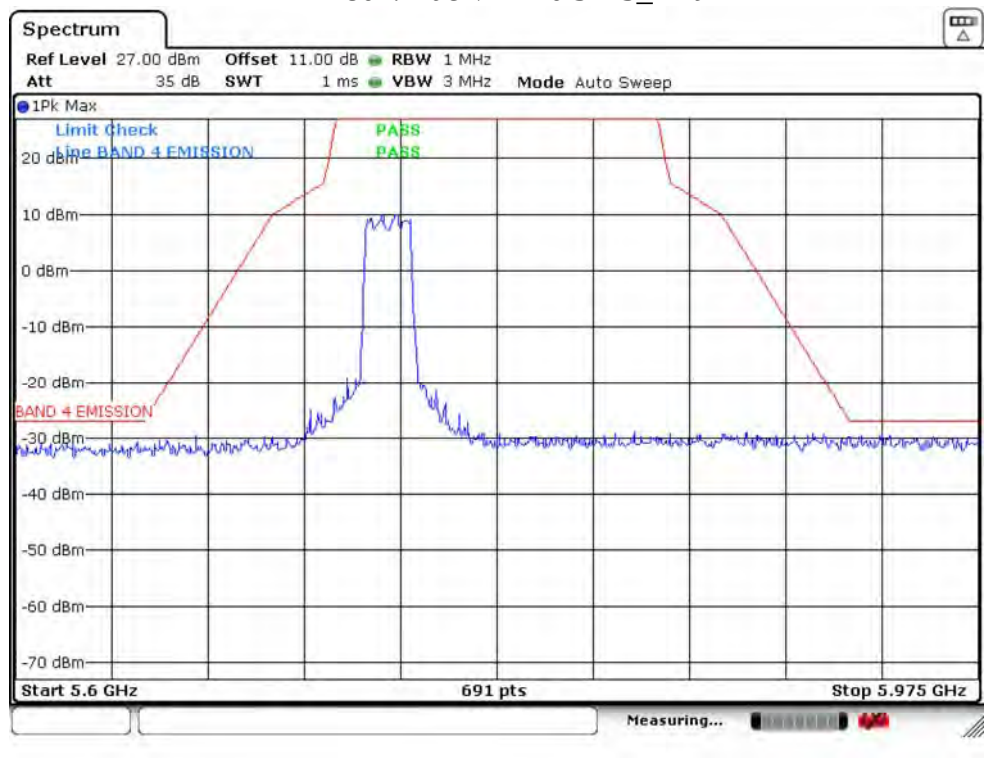
IEEE 802.11ac VHT20 5745_Ant 2
