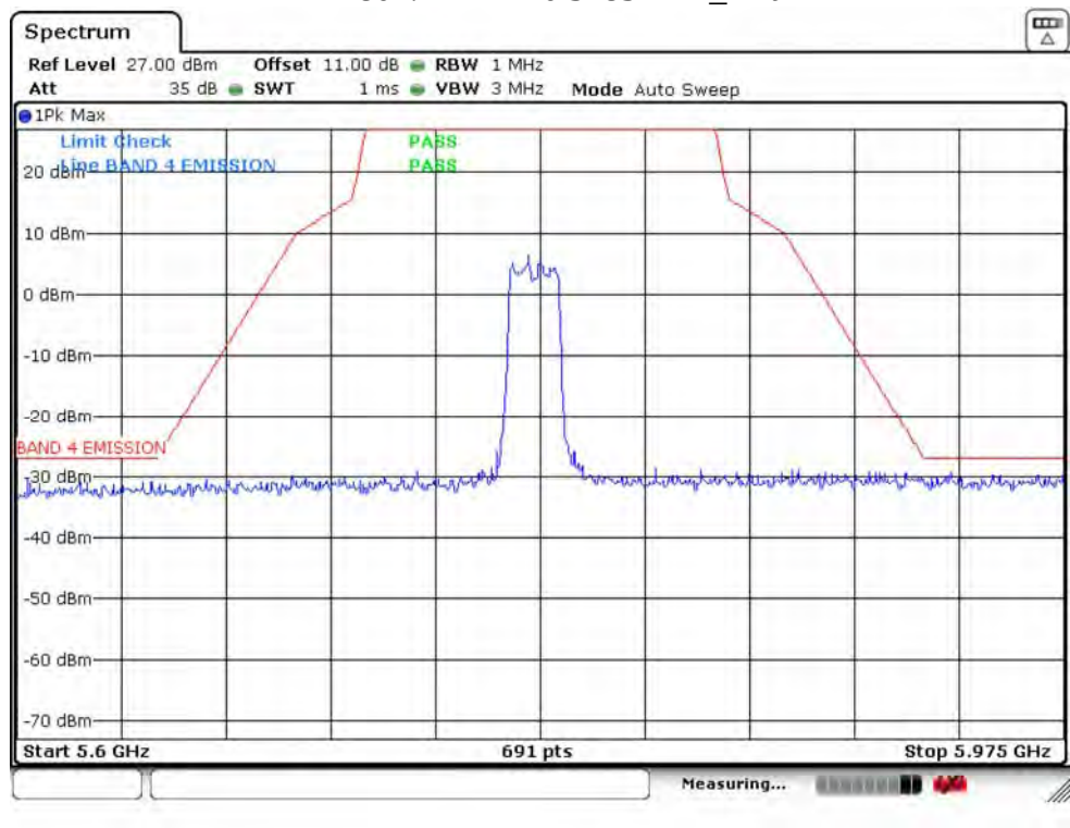
IEEE 802.11n HT20 5785MHz_Ant 1
