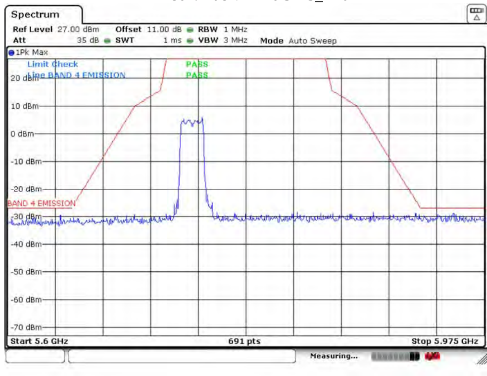
IEEE 802.11ac VHT20 5745_Ant 1
