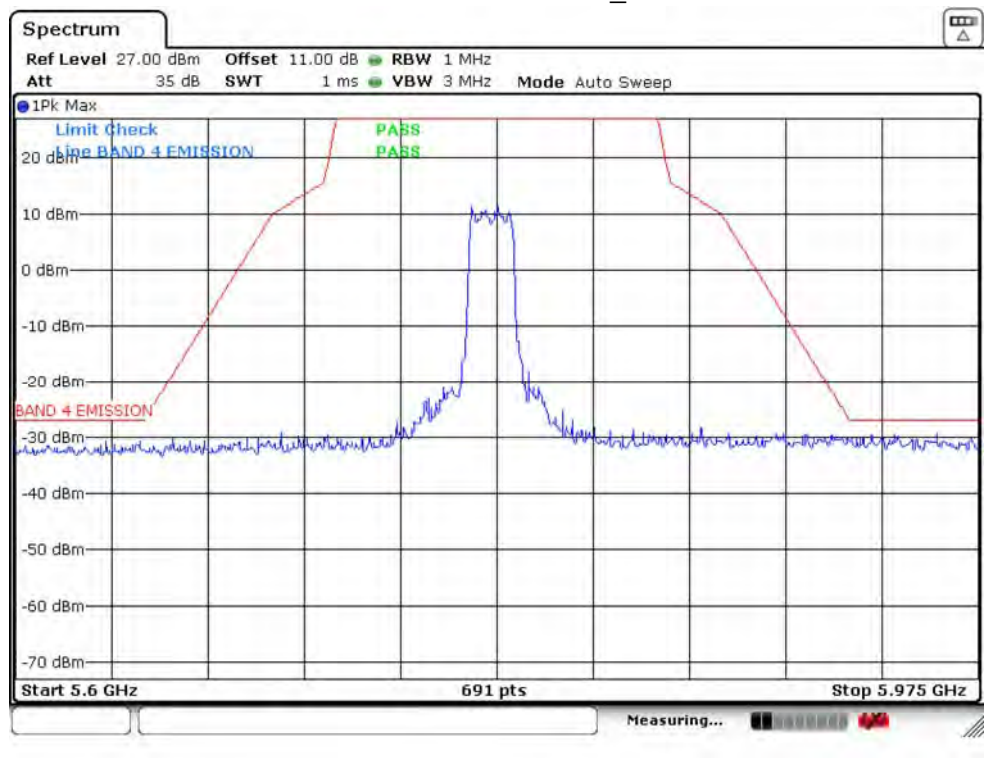
IEEE 802.11a 5785MHz_Ant 2
