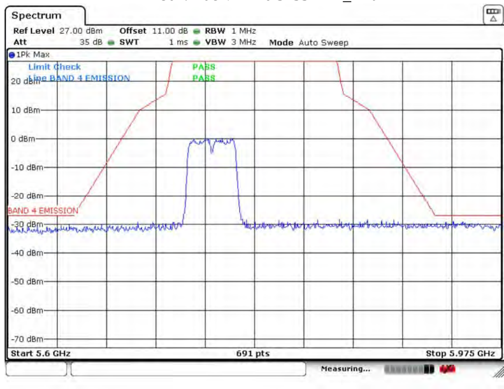
IEEE 802.11ac VHT40 5755MHz_Ant 1
