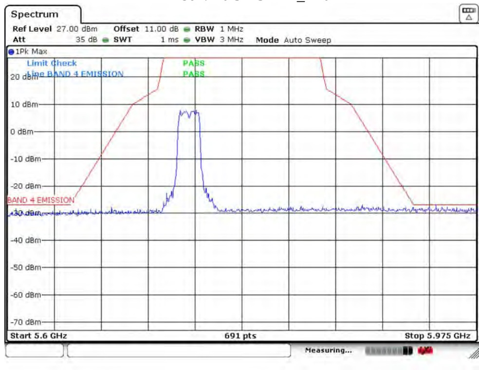
IEEE 802.11a 5745MHz_Ant 1
