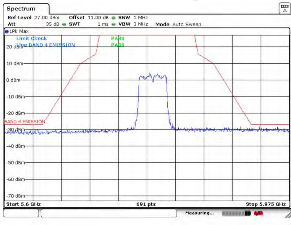
IEEE 802.11n HT40 5795MHz_Ant 1
