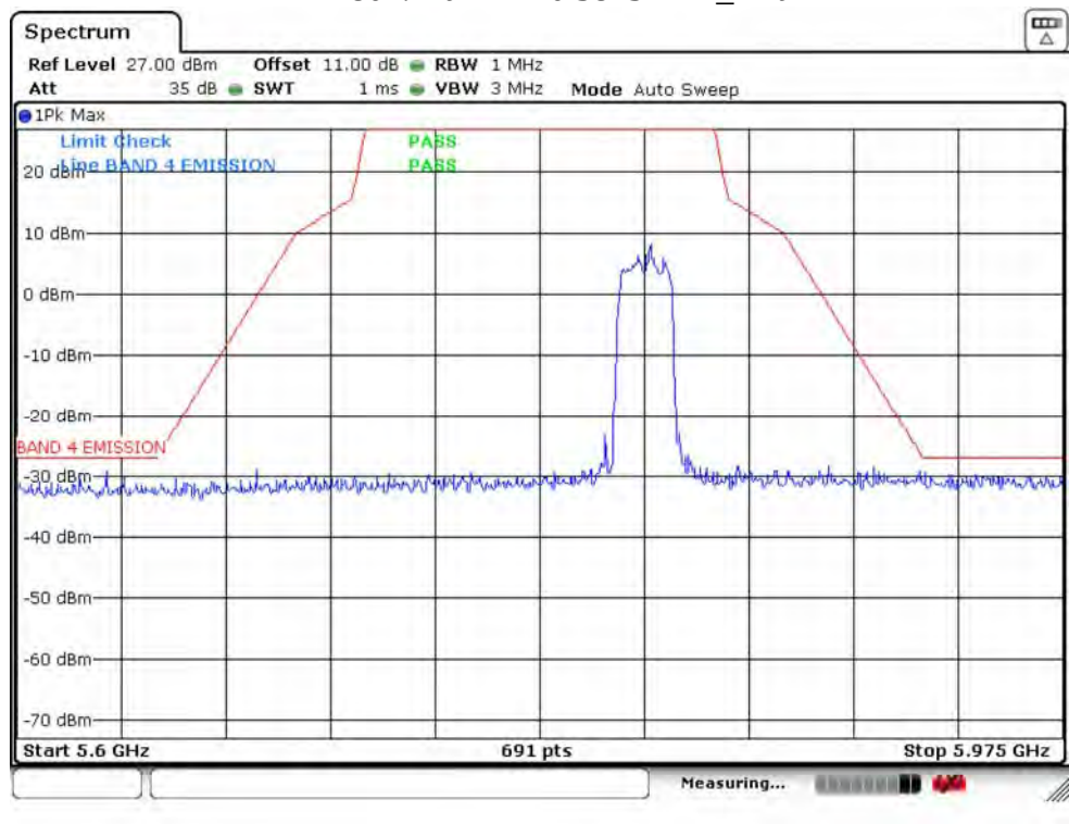
IEEE 802.11ax HE20 5825MHz_Ant 1
