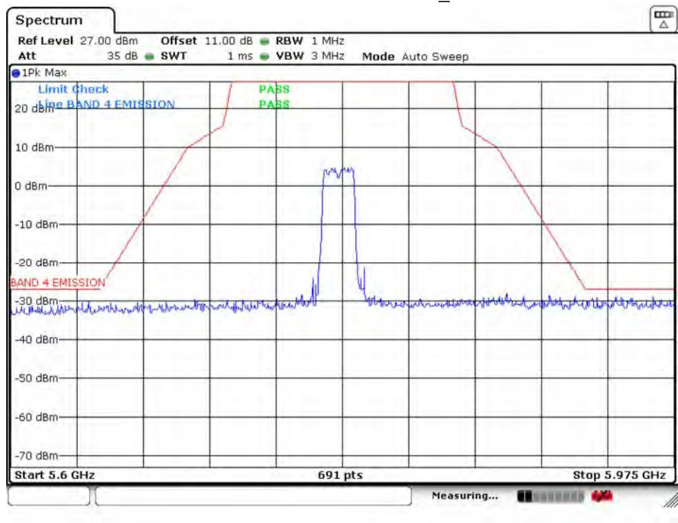
IEEE 802.11ac VHT20 5785_Ant 1
