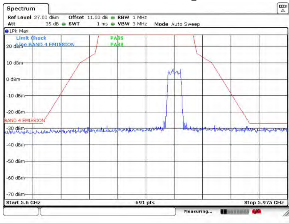
IEEE 802.11n HT20 5825MHz_Ant 1
