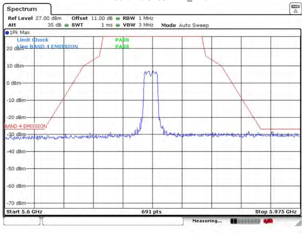
IEEE 802.11a 5785MHz_Ant 1
