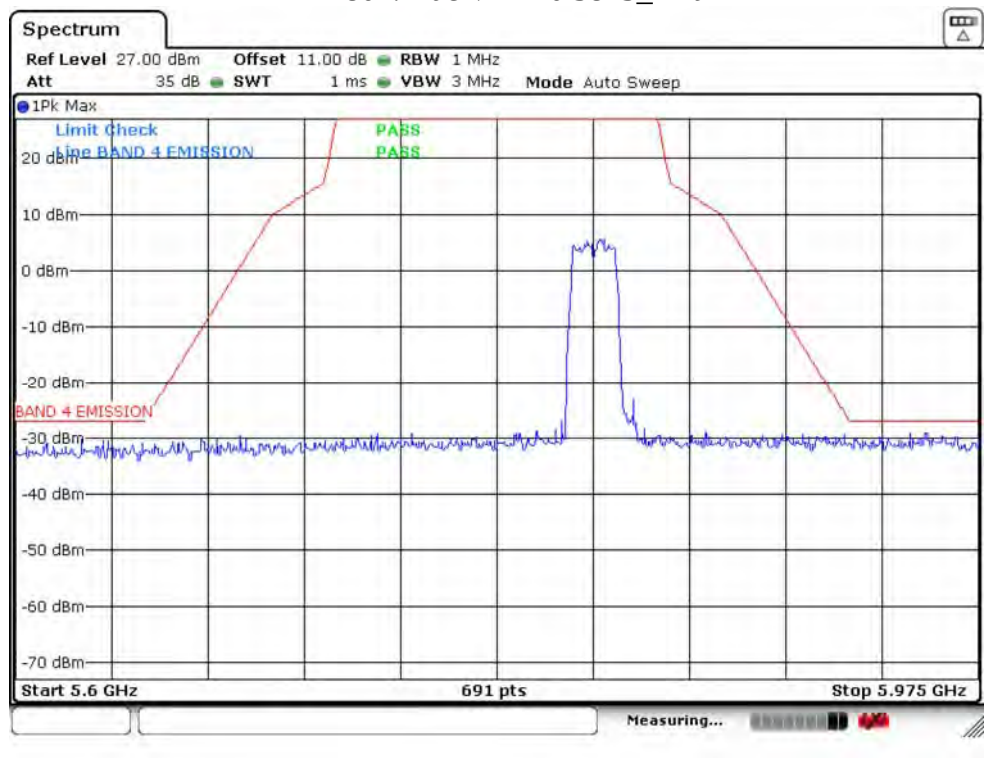
IEEE 802.11ac VHT20 5825_Ant 1
