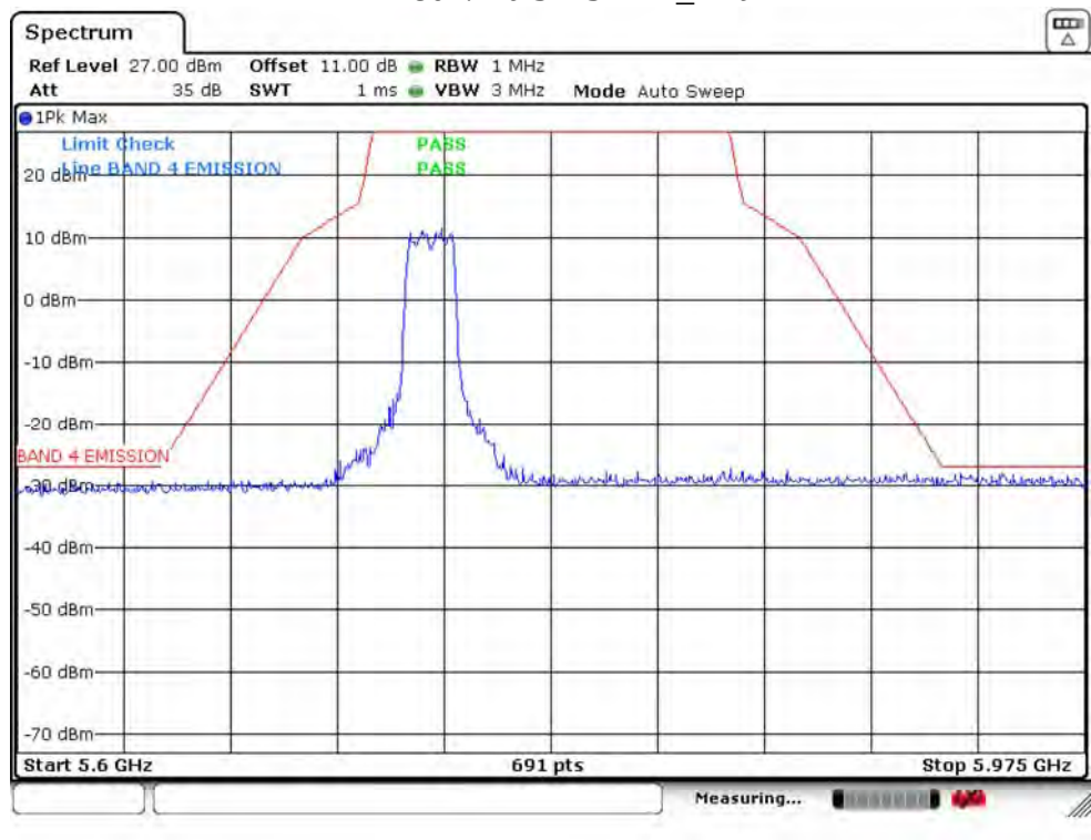
IEEE 802.11a 5745MHz_Ant 2
