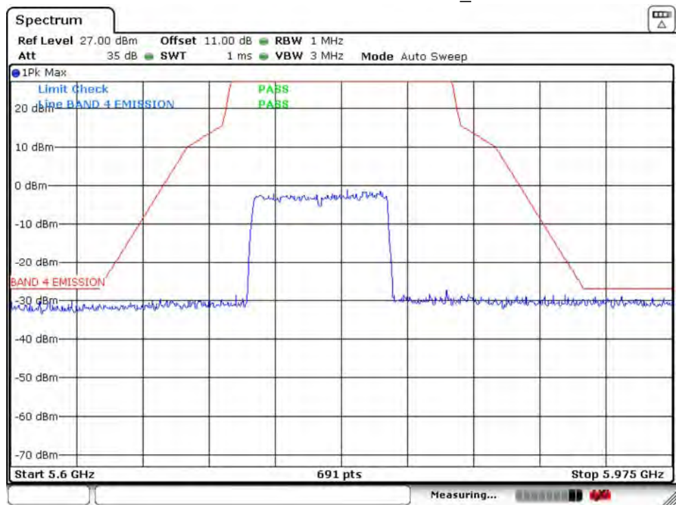
IEEE 802.11ac VHT80 5775MHz_Ant 1
