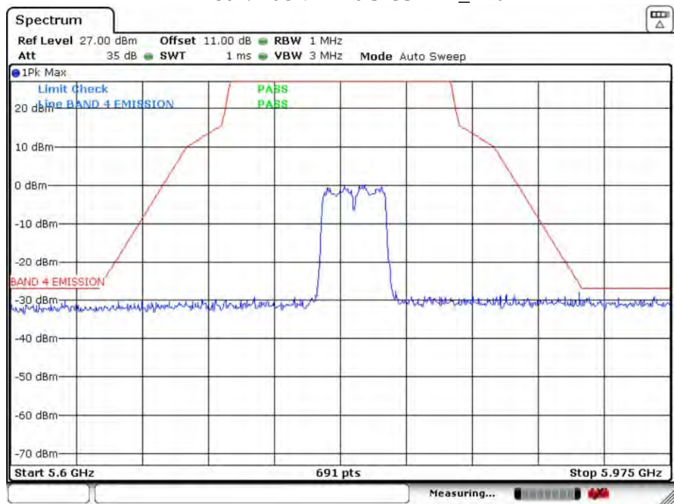
IEEE 802.11ac VHT40 5795MHz_Ant 1
