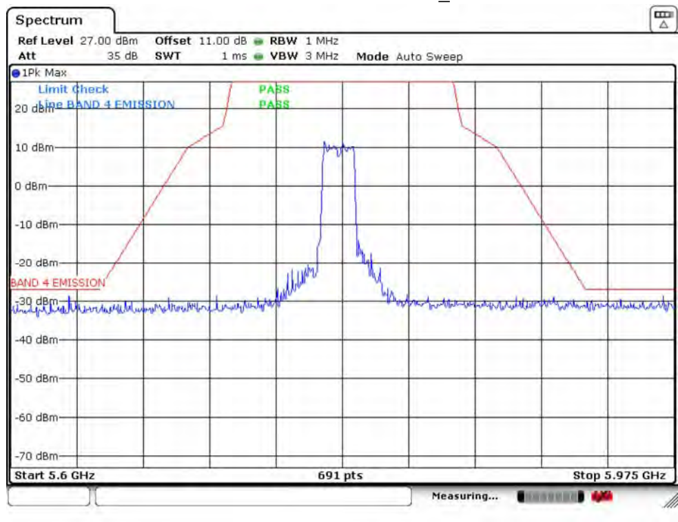
IEEE 802.11ac VHT20 5785_Ant 2
