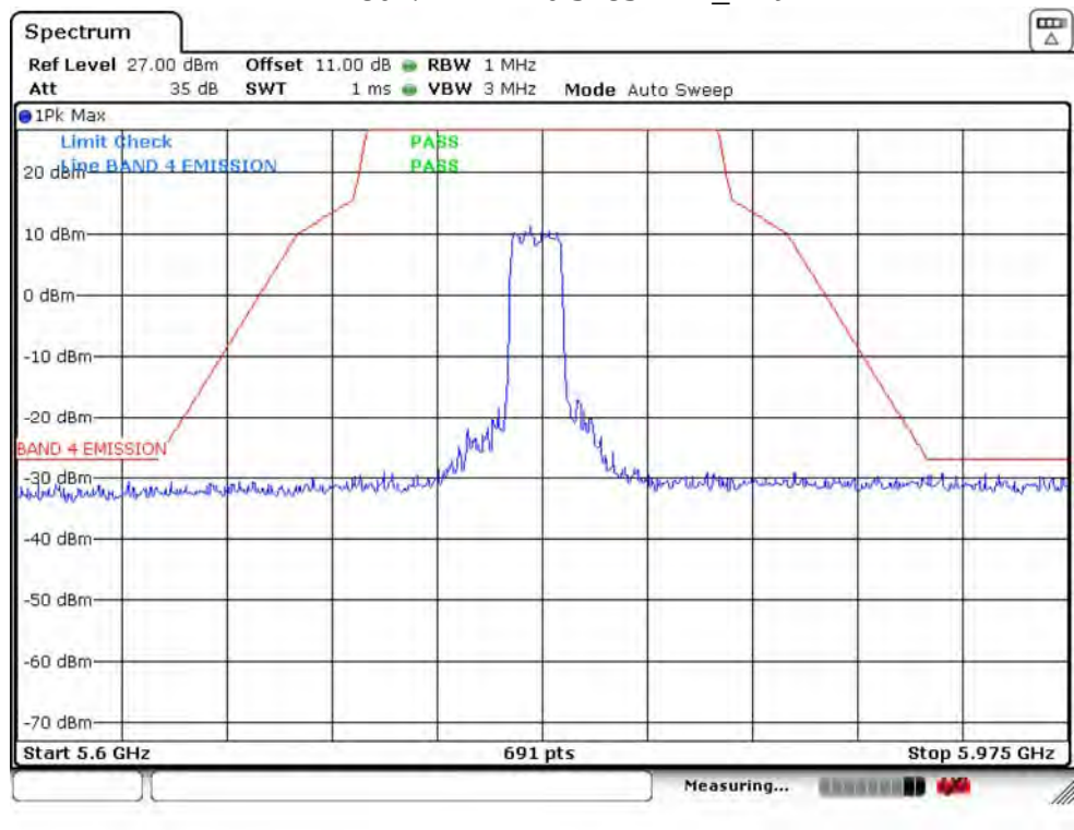
IEEE 802.11n HT20 5785MHz_Ant 2
