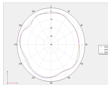
Theta 90 2D 图
