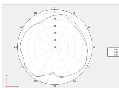
Phi 90 2D 图
