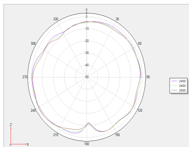
Phi 0 2D 图
