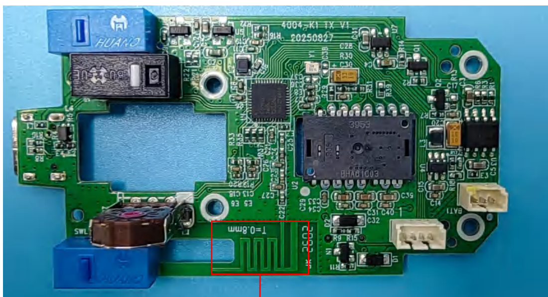
Antenna
