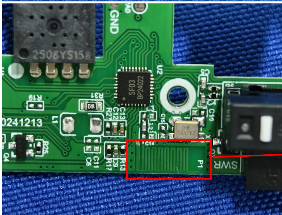
Antenna
