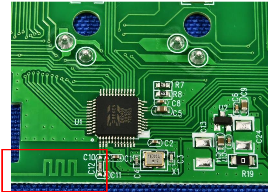
Antenna
