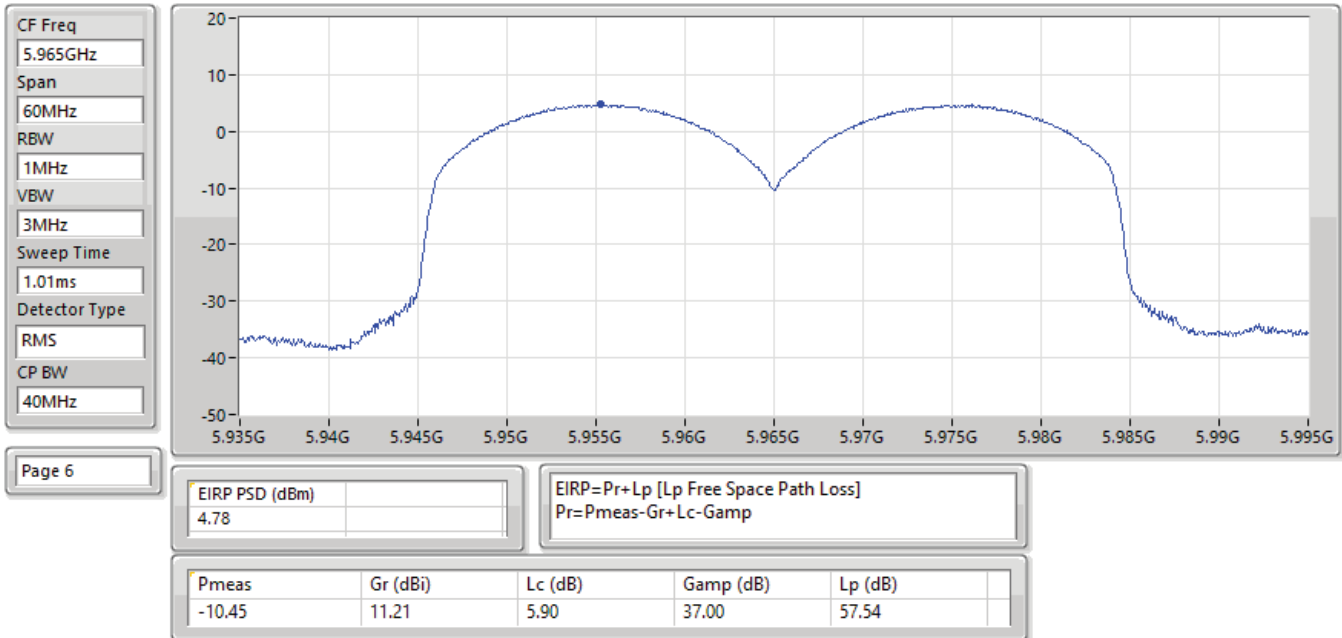
EIRP PSD;Band:6.2G;be40;BWch:40MHz;Nss:1,(M0);Nant:2;Ch:5965MHz;TX
