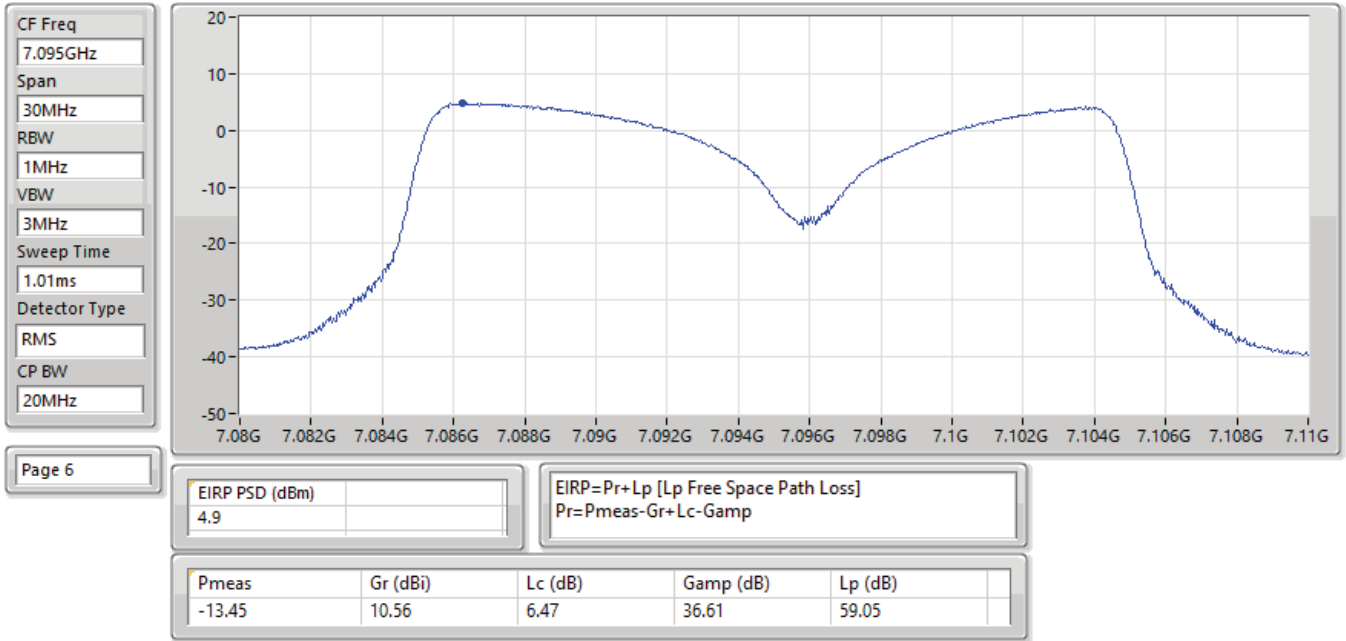
EIRP PSD;Band:7.0G;be20;BWch:20MHz;Nss:1,(M0);Nant:2;Ch:7095MHz;TX
