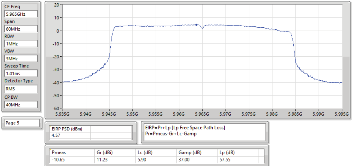
EIRP PSD;Band:6.2G;be40,BF;BWch:40MHz;Nss:1,(M0);Nant:2;Ch:5965MHz;TX
