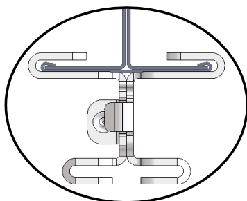
5/16" T-Bar
