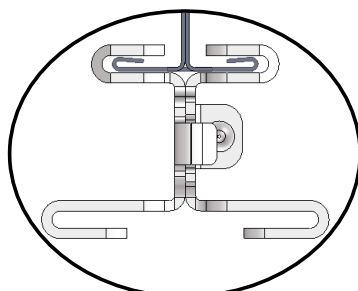
9/16" T-Bar
