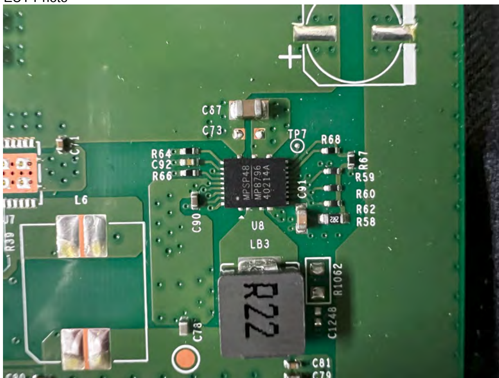
(64) EUT Photo
