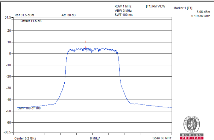
802.11ax (HE20) / Chain 2 : CH 40
