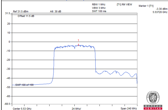
802.11ax (HE80+HE80) / Chain 0 : CH 106+122(L)
