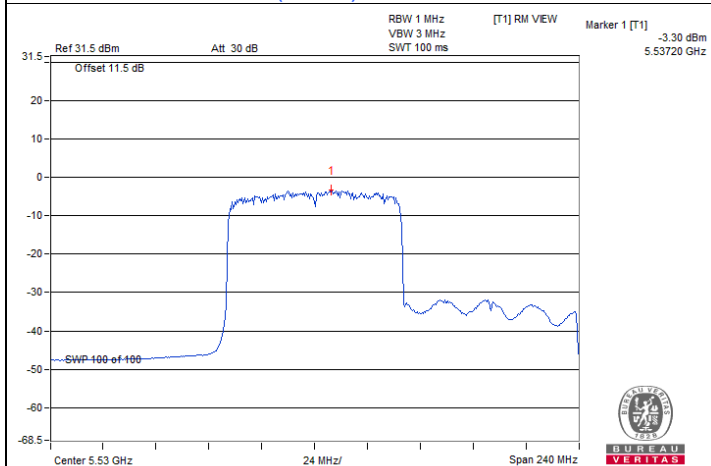
802.11ax (HE80+HE80) / Chain 0 : CH 106+122(L)
