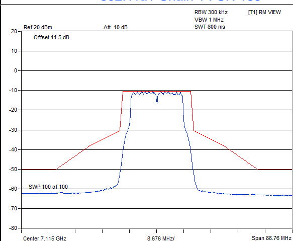
802.11a / Chain 1 : CH 233
