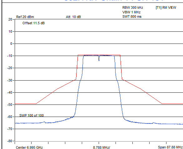
802.11a / Chain 1 : CH 209
