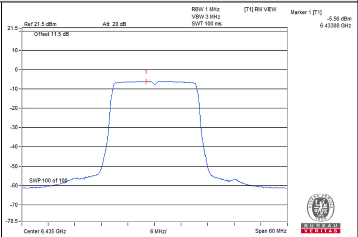
802.11ax (HE20) / Chain 0 : CH 97
