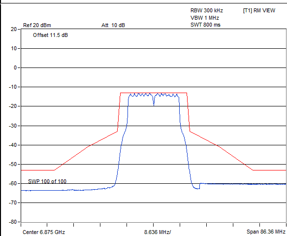
802.11a / Chain 1 : CH 185
