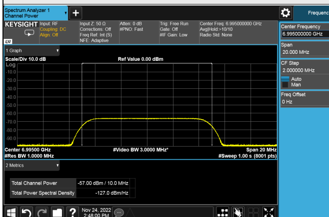
802.11ax (HE20) / CH 209
