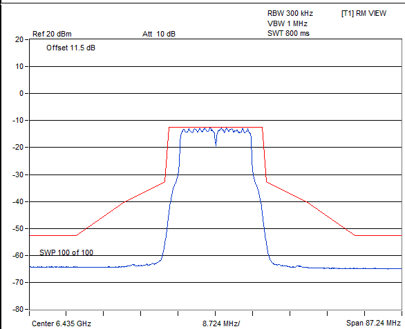
802.11a / Chain 1 : CH 97
