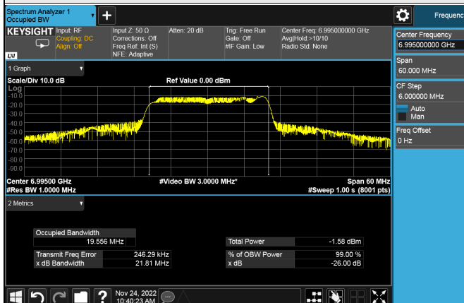
802.11ax (HE20) / CH 209
