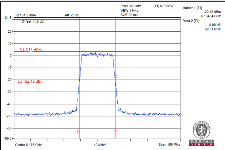
802.11ax (HE20) / Chain 0 : CH 45
