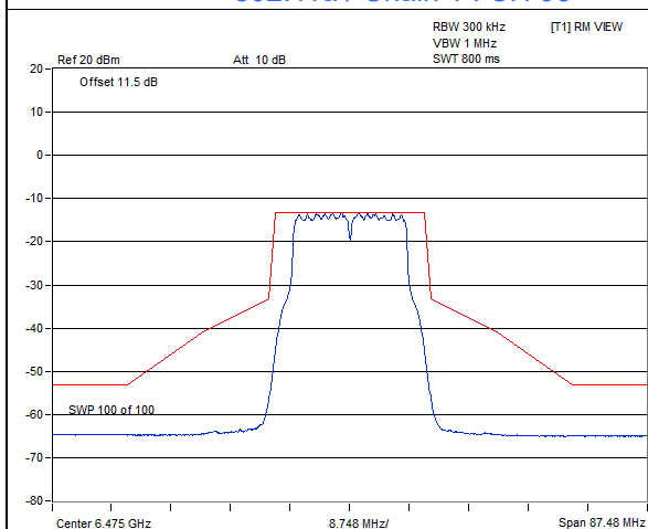
802.11a / Chain 1 : CH 105
