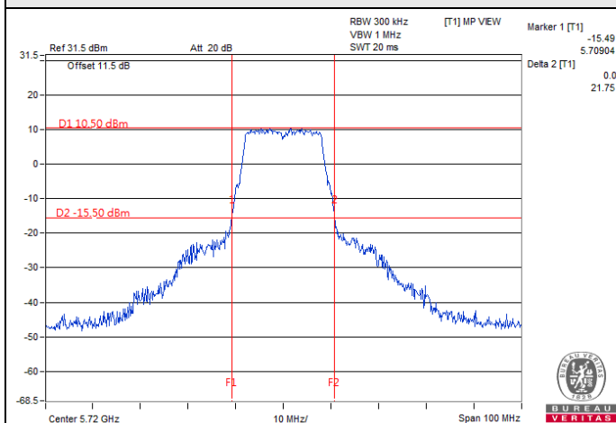
802.11a / Chain 0 : CH 144 (U-NII-2C)
