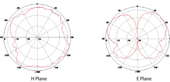
Port 3: 5500MHz
