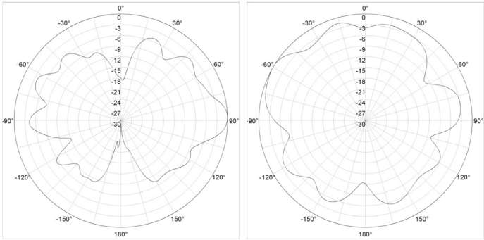
E-Plane Pattern H-Plane Pattern 6 GHz
