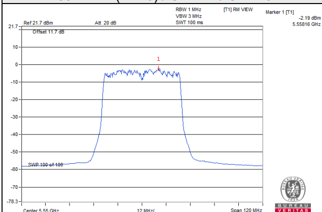
802.11ax (HE80+80) / Chain 1 / CH 106+122
