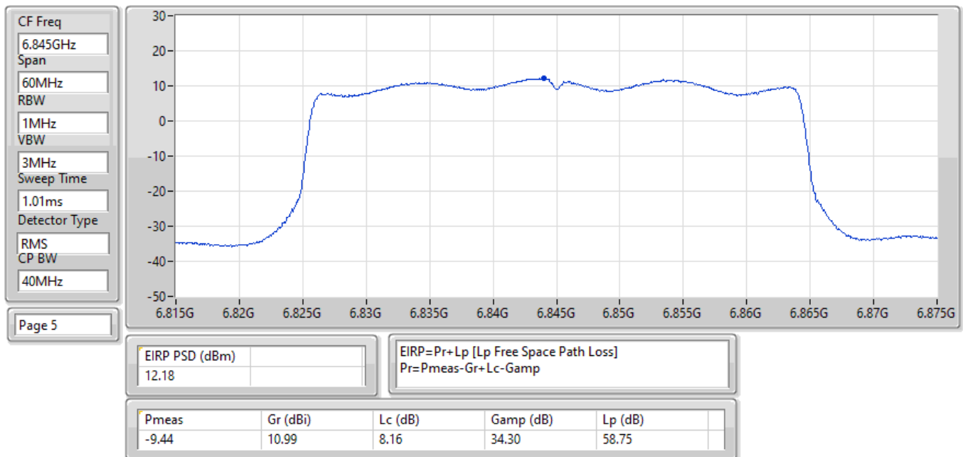
EIRP PSD;Band:6.7G;ax40;BWch:40MHz;Nss:1,(M0);Nant:2;Ch:6845MHz;TX
