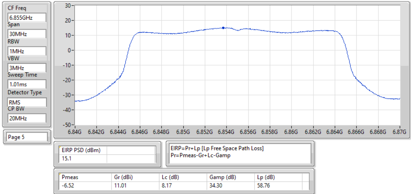
EIRP PSD;Band:6.7G;ax20;BWch:20MHz;Nss:1,(M0);Nant:2;Ch:6855MHz;TX
