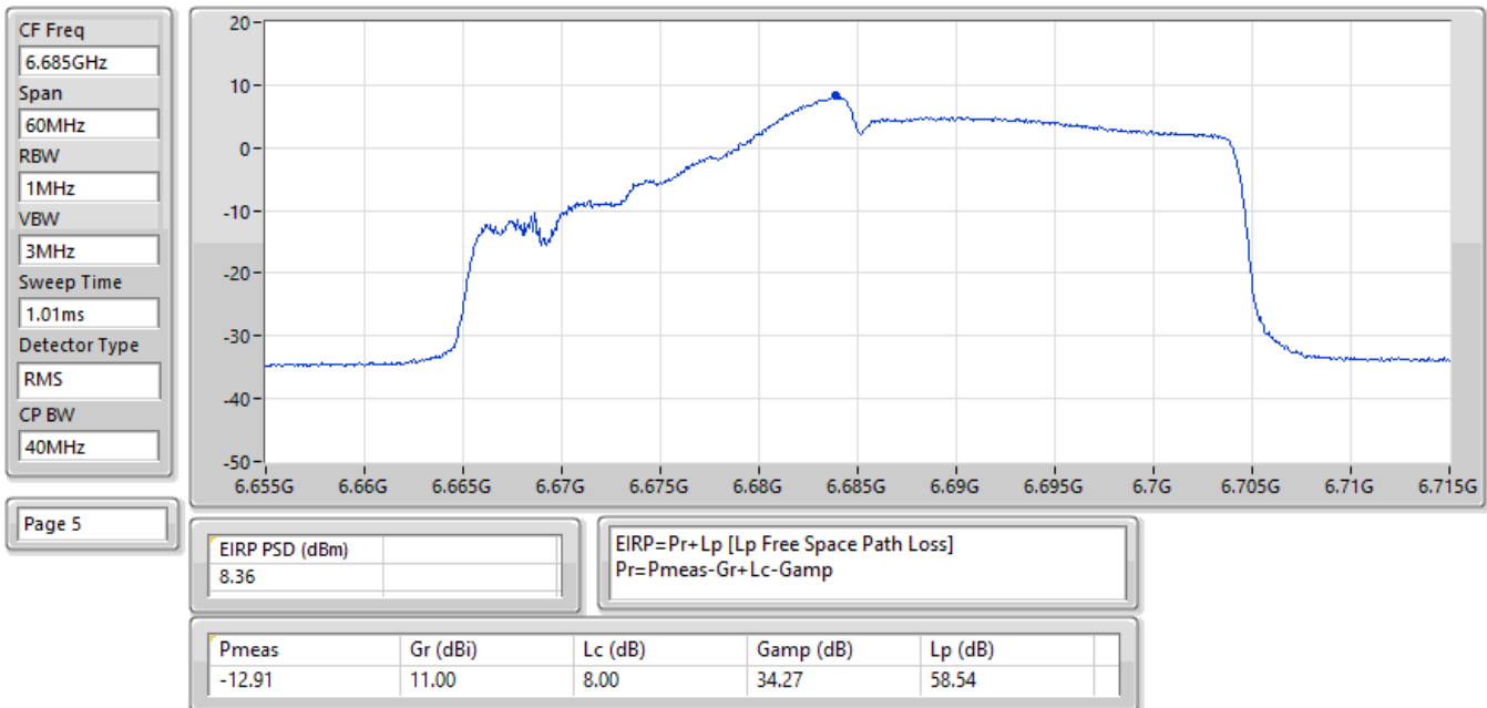
EIRP PSD;Band:6.7G;ax40,BF;BWch:40MHz;Nss:1,(M0);Nant:2;Ch:6685MHz;TX
