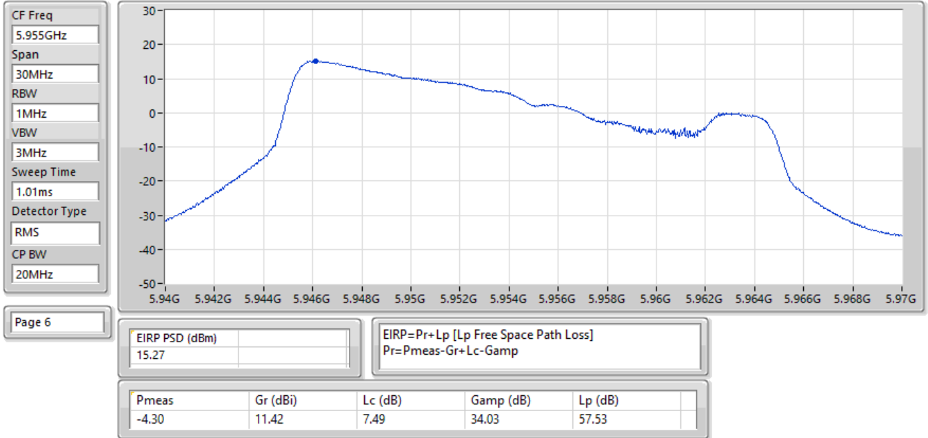
EIRP PSD;Band:6.2G;ax20,BF;BWch:20MHz;Nss:1,(M0);Nant:2;Ch:5955MHz;TX
