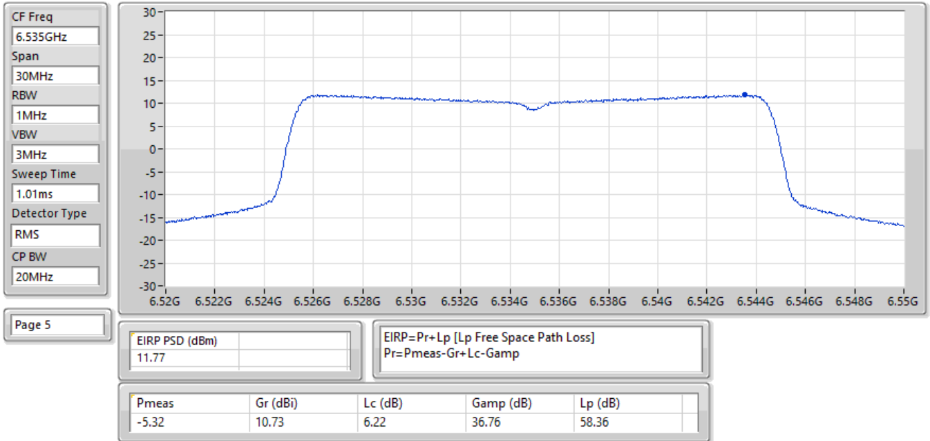
EIRP PSD;Band:6.7G;ax20,BF;BWch:20MHz;Nss:1,(M0);Nant:4;Ch:6535MHz;TX
