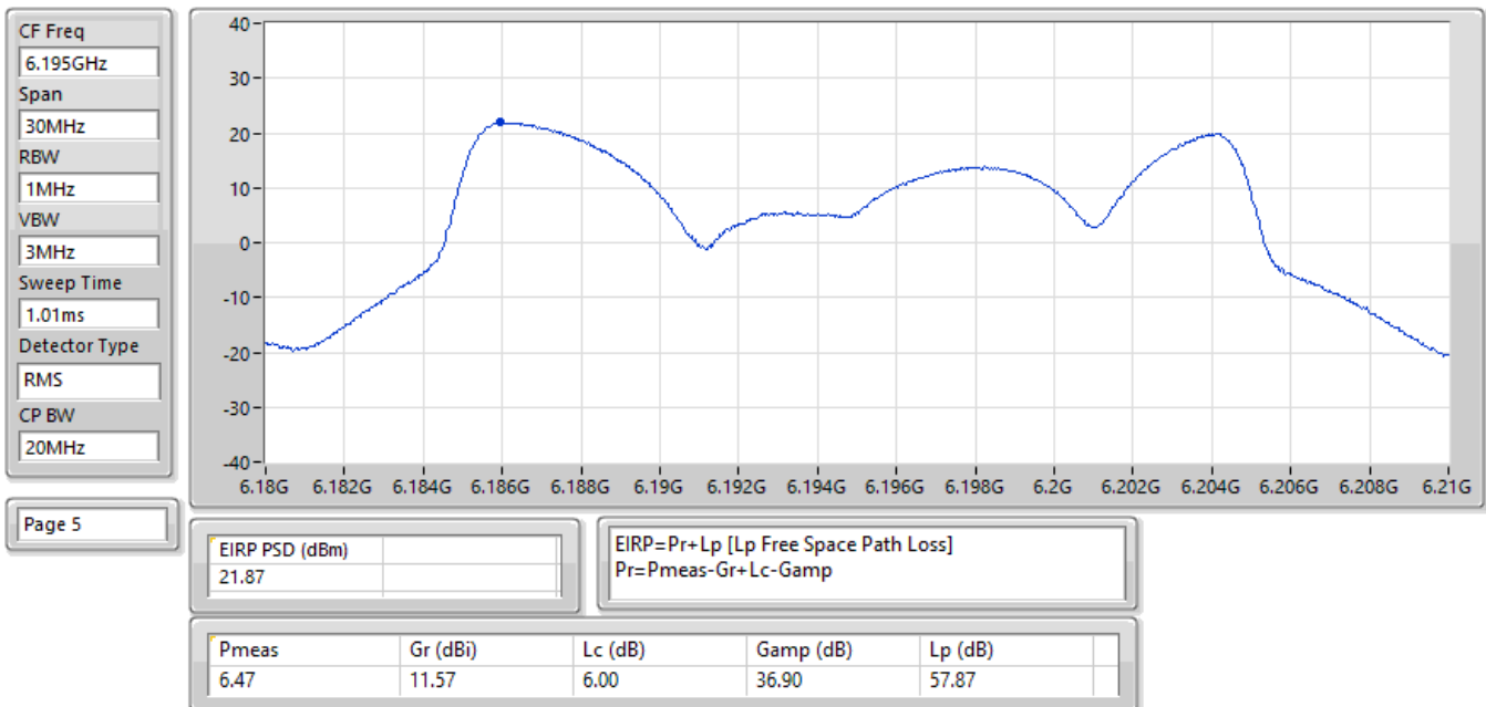
EIRP PSD;Band:6.2G;ax20;BWch:20MHz;Nss:1,(M0);Nant:4;Ch:6195MHz;TX
