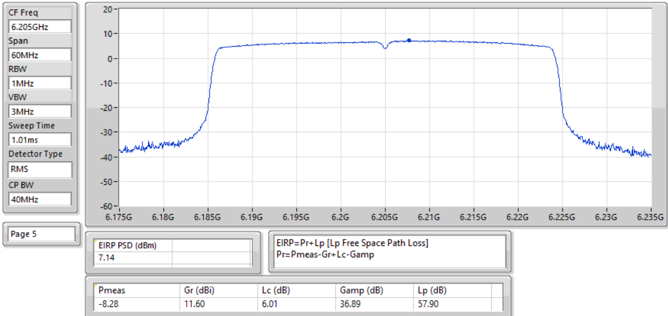
EIRP PSD;Band:6.2G;ax40,BF;BWch:40MHz;Nss:1,(M0);Nant:4;Ch:6205MHz;TX
