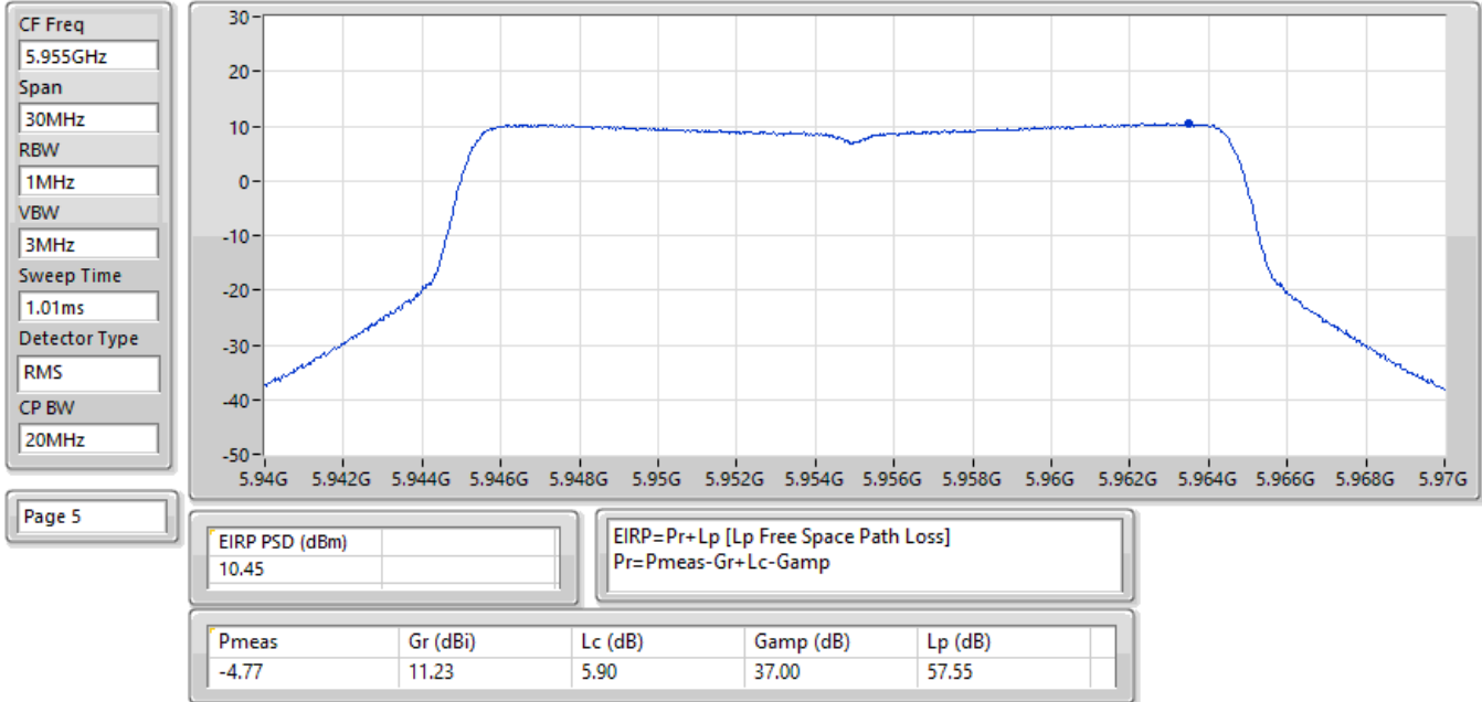
EIRP PSD;Band:6.2G;ax20,BF;BWch:20MHz;Nss:1,(M0);Nant:4;Ch:5955MHz;TX
