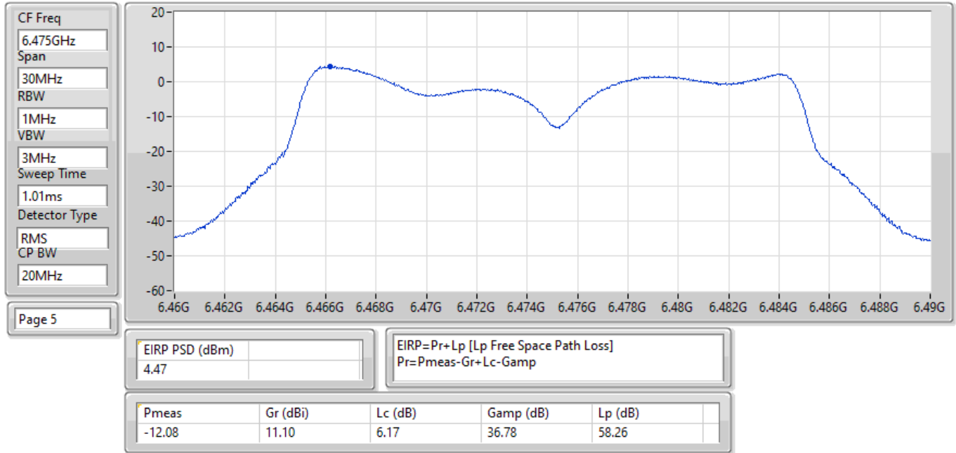
EIRP PSD;Band:6.4G;be20;BWch:20MHz;Nss:1,(M0);Nant:4;Ch:6475MHz;TX
