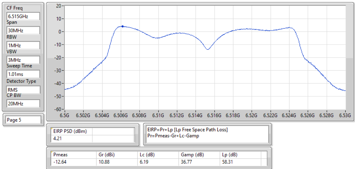
EIRP PSD;Band:6.4G;be20;BWch:20MHz;Nss:1,(M0);Nant:4;Ch:6515MHz;TX
