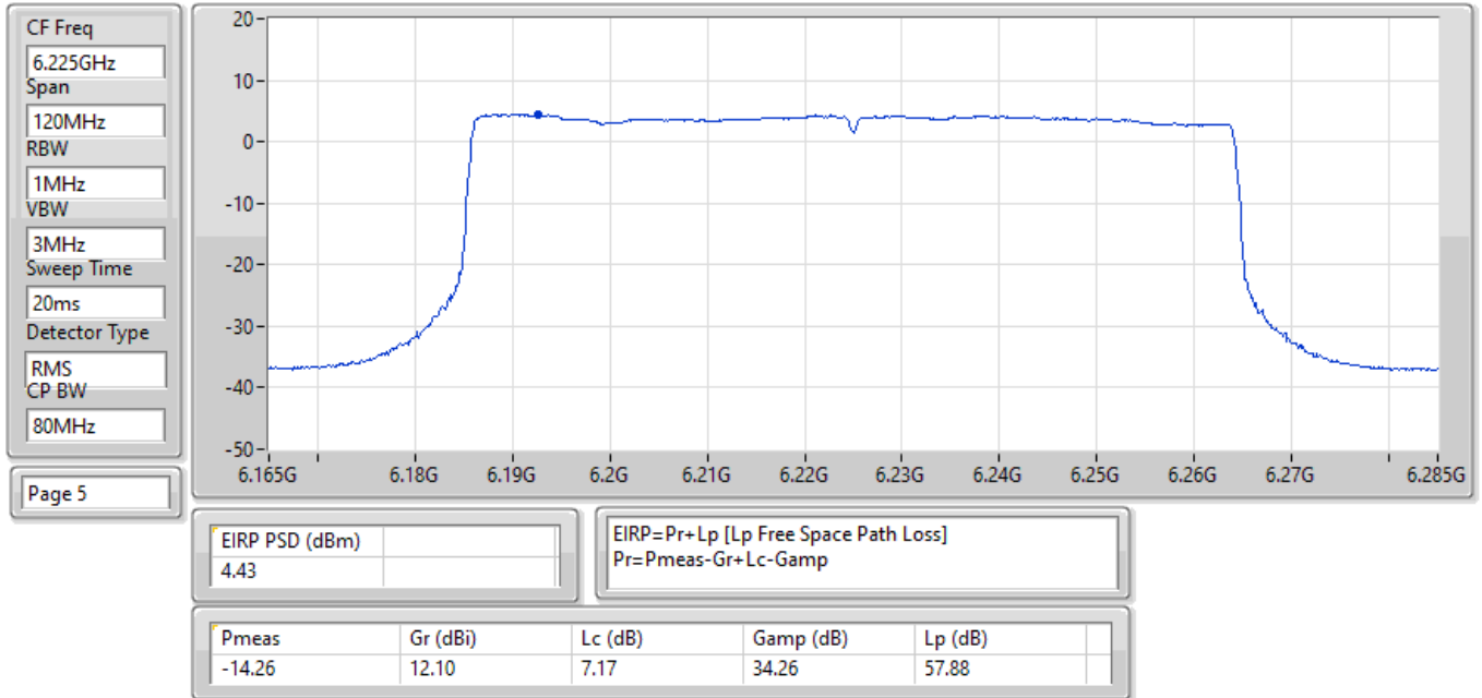
EIRP PSD;Band:6.2G;be80,BF;BWch:80MHz;Nss:1,(M0);Nant:4;Ch:6225MHz;TX
