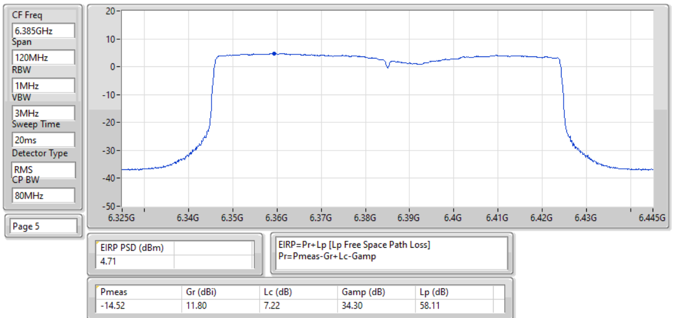
EIRP PSD;Band:6.2G;be80,BF;BWch:80MHz;Nss:1,(M0);Nant:4;Ch:6385MHz;TX
