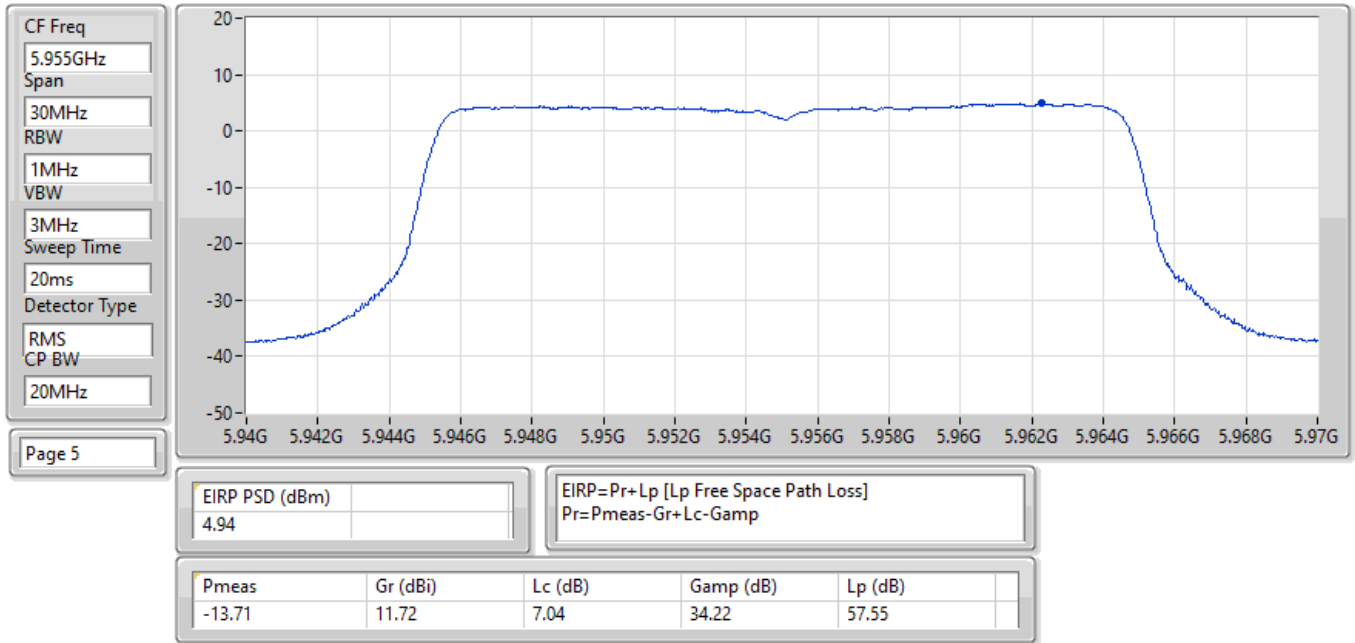
EIRP PSD;Band:6.2G;be20,BF;BWch:20MHz;Nss:1,(M0);Nant:4;Ch:5955MHz;TX
