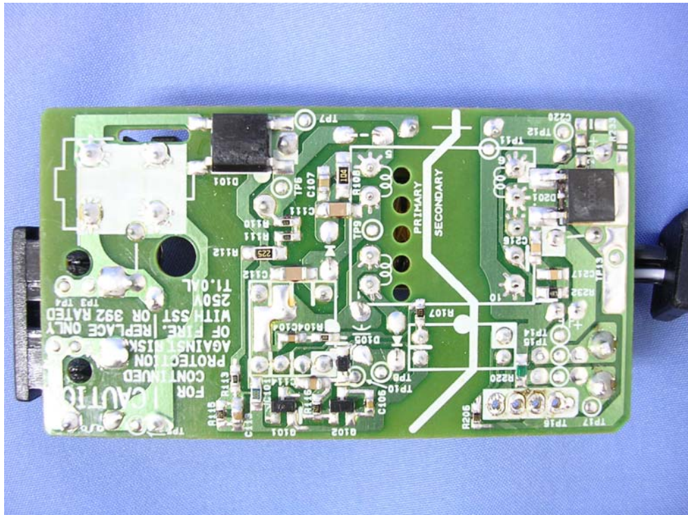
(54) EUT Photo
