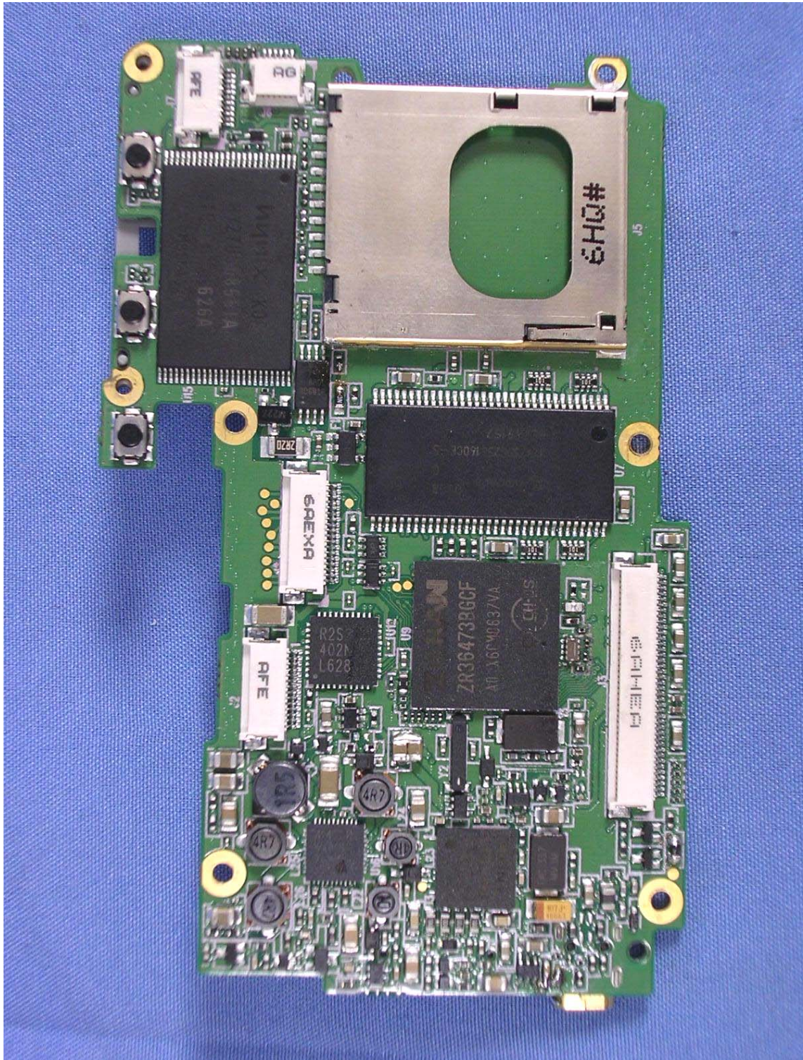
(36) EUT Photo
