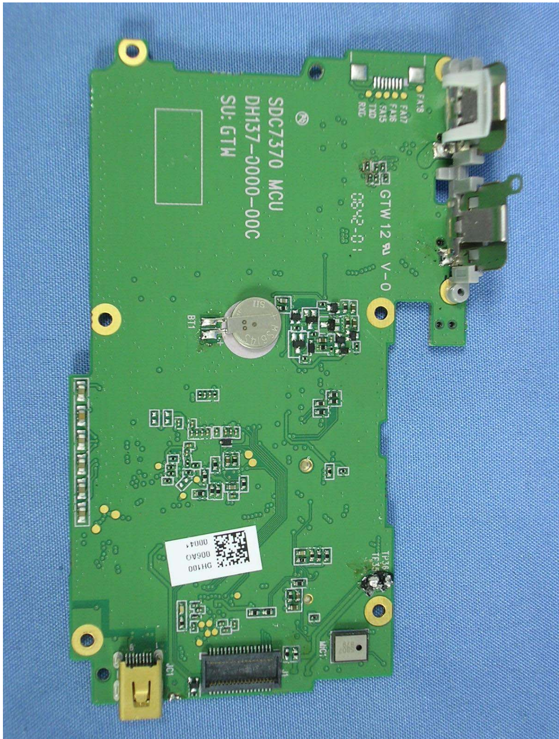
(37) EUT Photo
