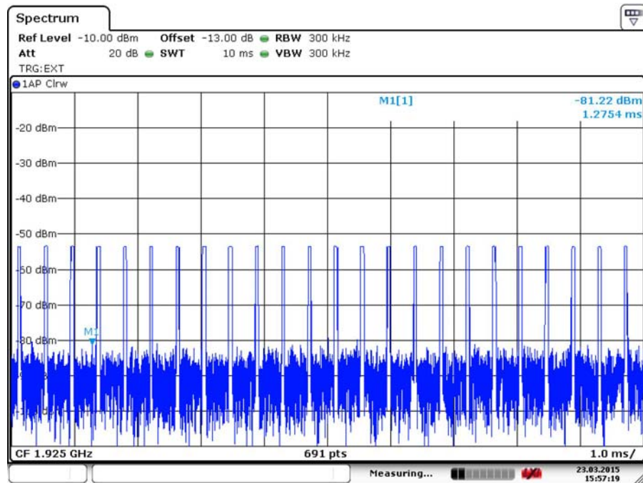
50 µs Pulses
