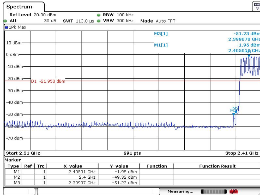
(Plot 4.5.2.1 A: Hopping Mode @ GFSK)
