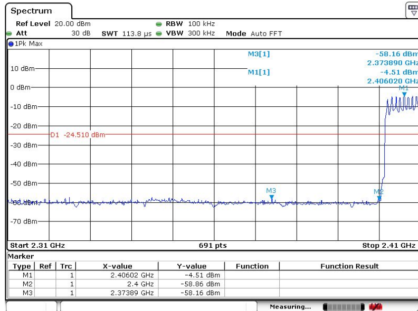
(Plot 4.5.2.2 A: Hopping Mode @ 8DPSK)
