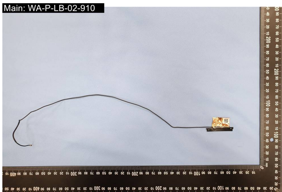
EUT Photo (10)
