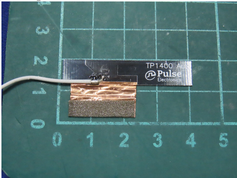
(33) EUT Photo_Pulse Aux Antenna
