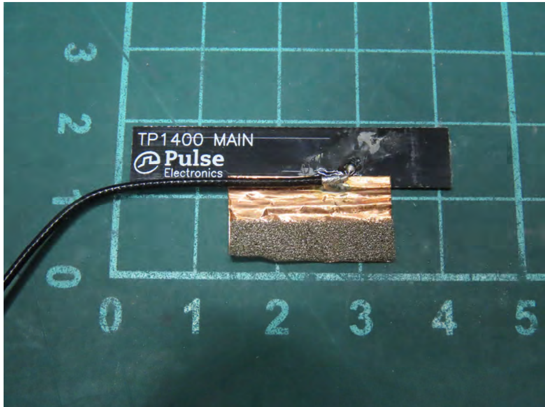
(33) EUT Photo
