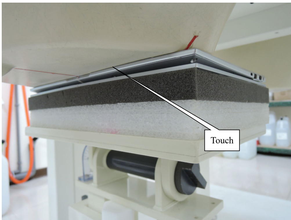
EUT Back(PAD)
